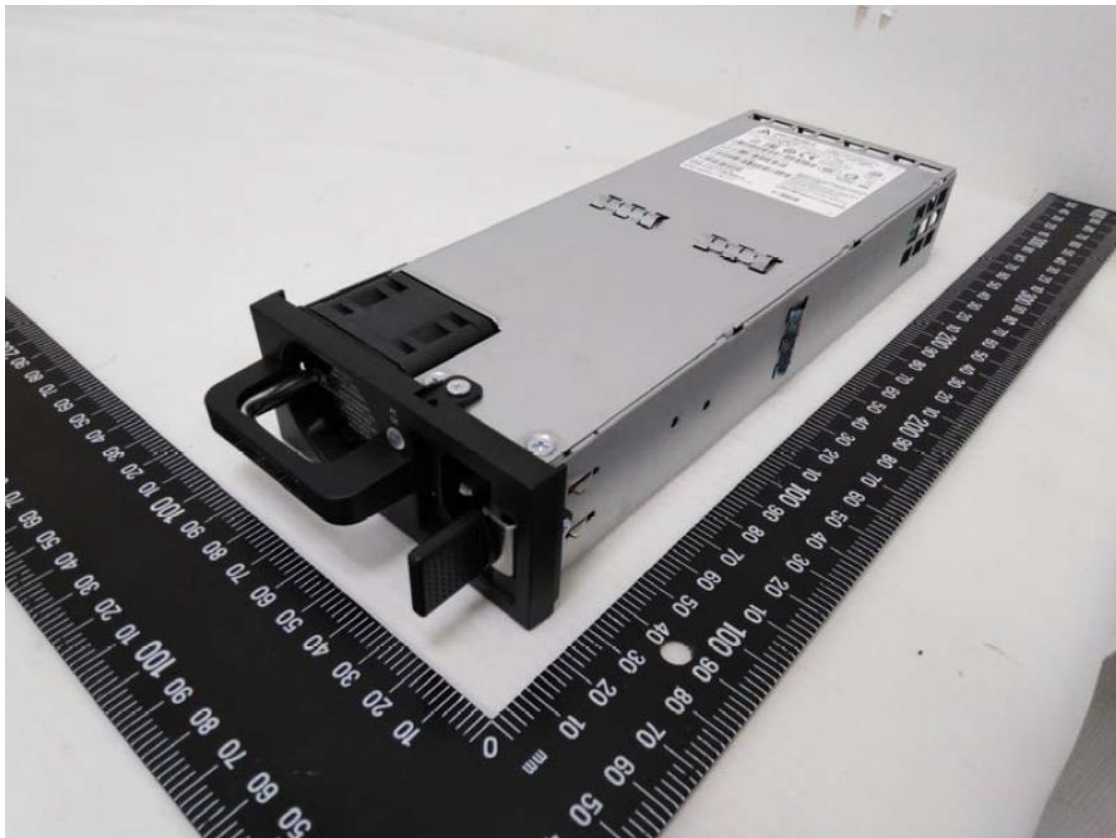
交流電源供應器-正視圖
