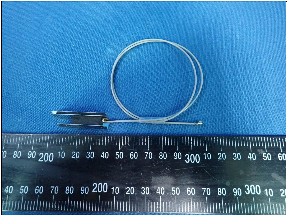
Antenna - Model: ADM205G37C1
