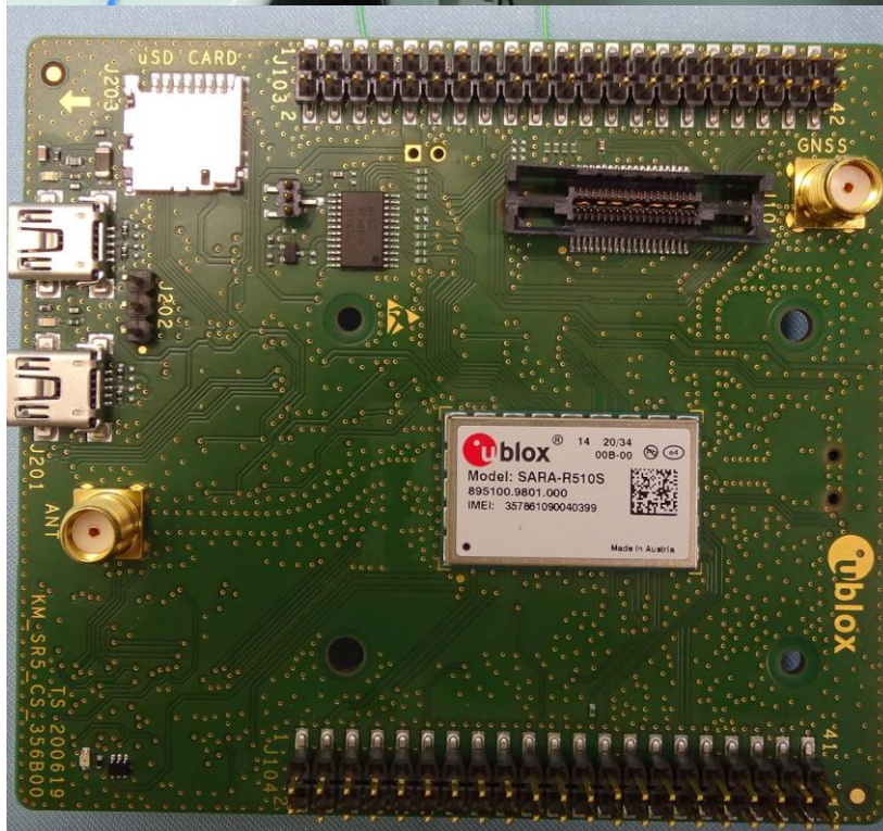
EUT 近照
