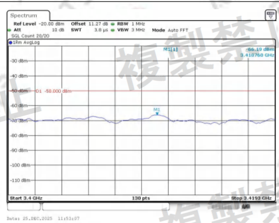
3400.0-3419.3_new Band 3 5MHz/1747.5/Mid QPSK 1@0
