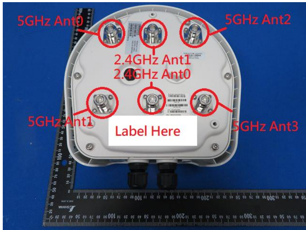
(1) EUT Photo (APEX0574)
