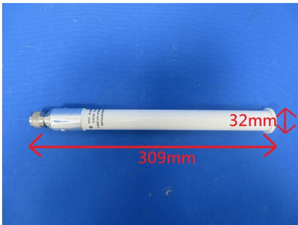
(8) EUT Photo (ANT-2X2-2005-Vpol)
