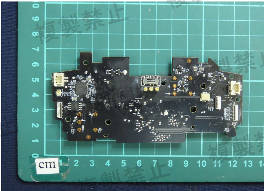
(44) EUT Photo
