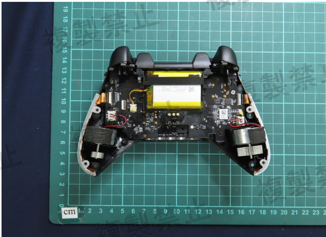
(36) EUT Photo
