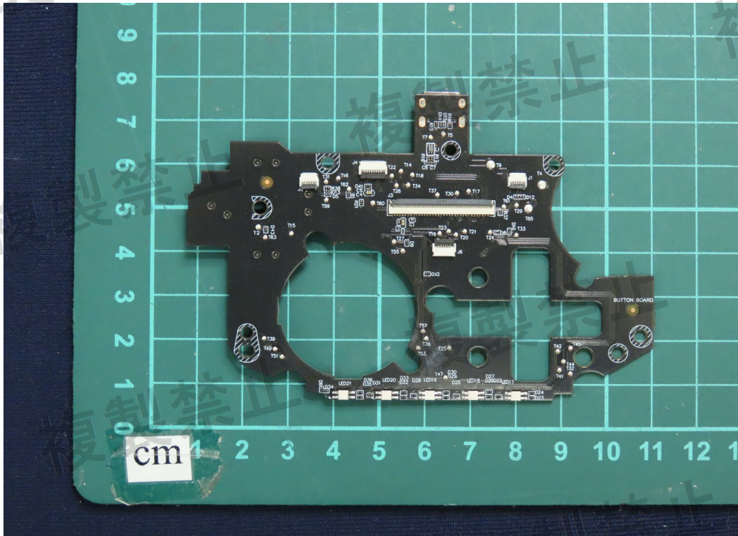
(60) EUT Photo
