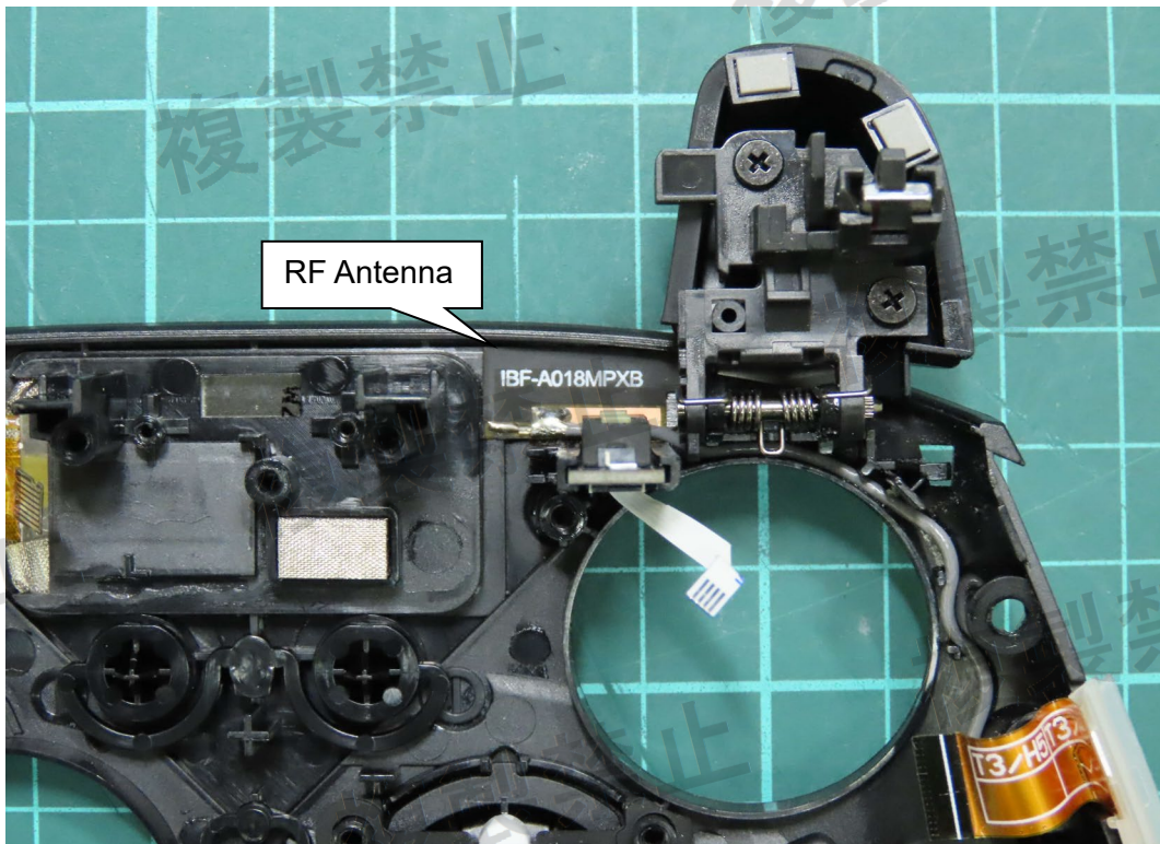
(70) EUT Photo
