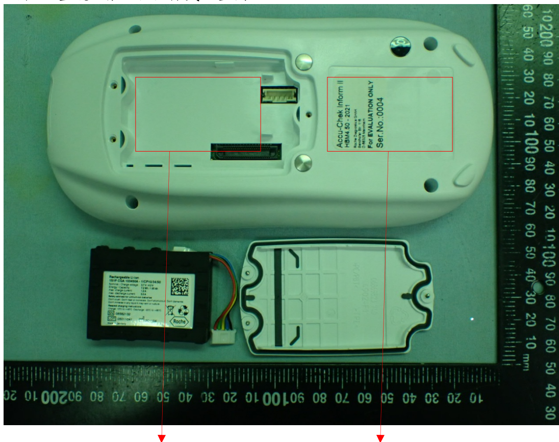
照片20 型號&amp;審驗合格標籤示意圖
