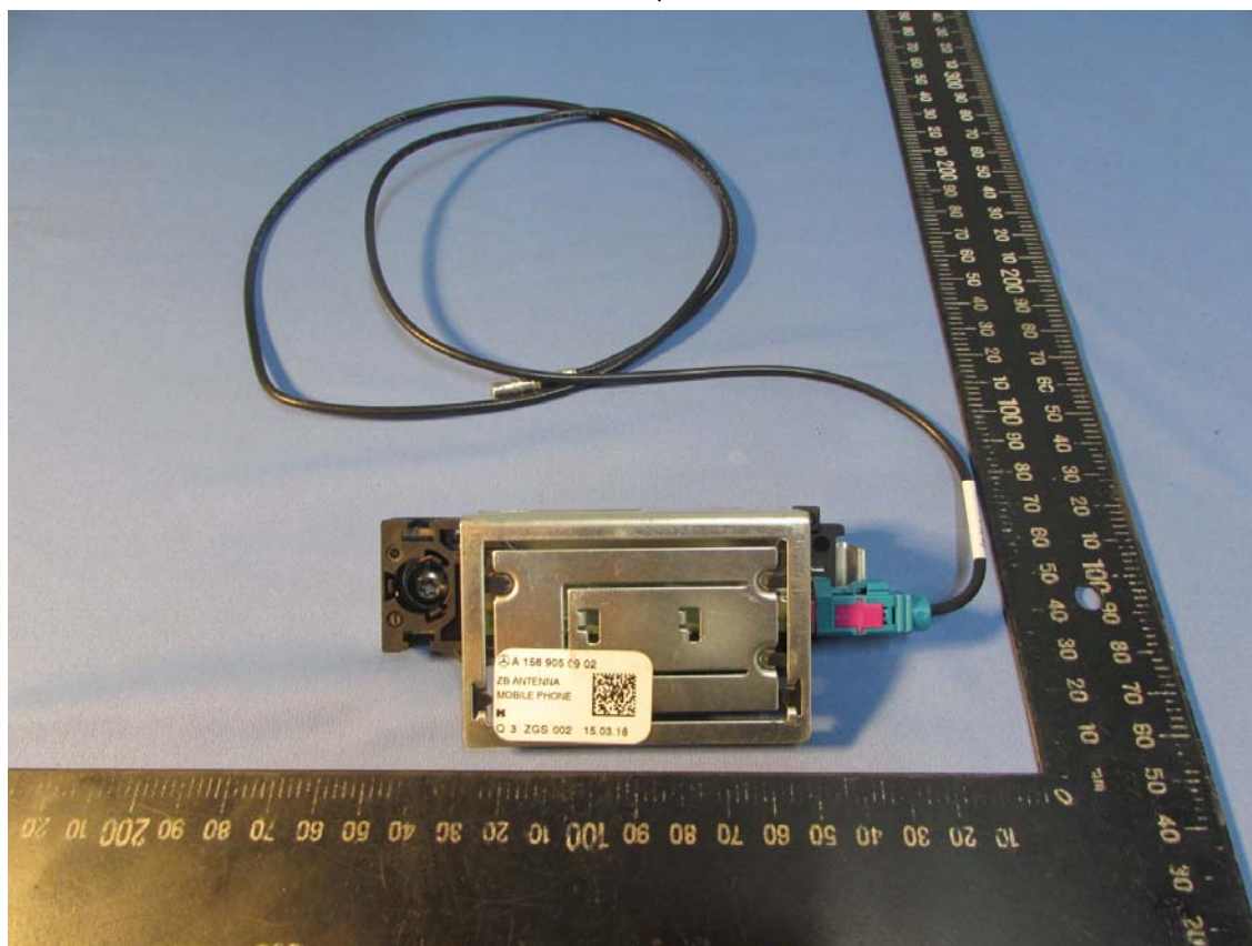
LTE天線-背面照
