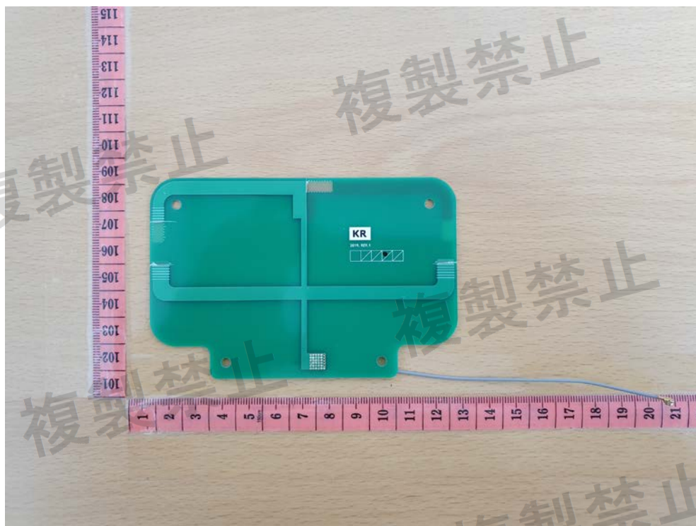
RFID Antenna 1 (M/N: MYA SPS-997)
