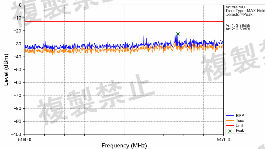
802.11be(EHT40)_LCH_5510MHz_RU484_Left_MIMO_NTNV
