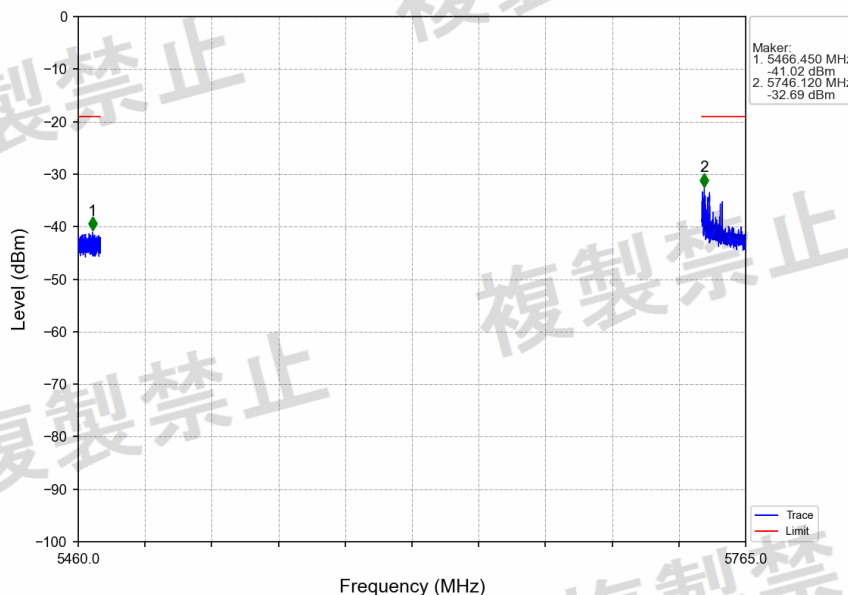
802.11ac(VHT20)_HHCH_5720MHz_Ant2_NTNV
