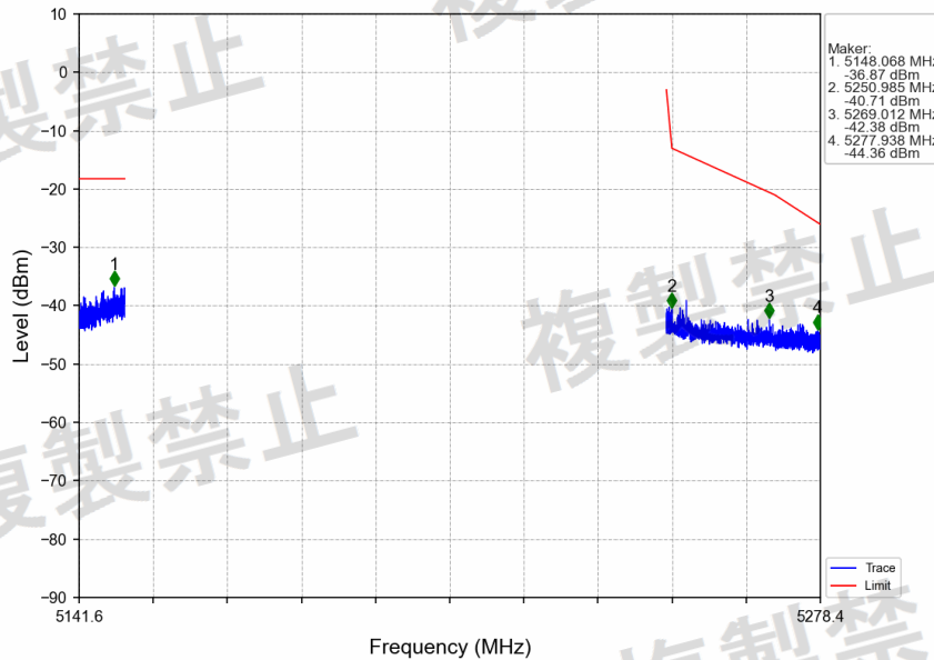
802.11be(EHT40)_LCH_5190MHz_RU484_Left_Ant2_NTNV
