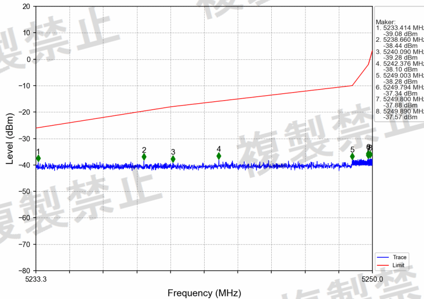
802.11be(EHT20)_MCH_5300MHz_RU242_Left_MIMO_NTNV
