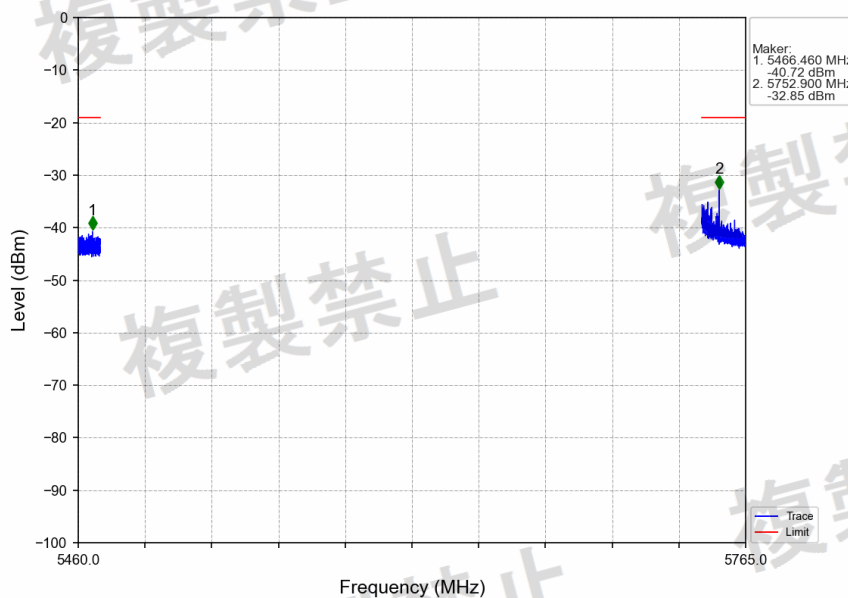
802.11ac(VHT20)_HHCH_5720MHz_Ant2_NTNV
