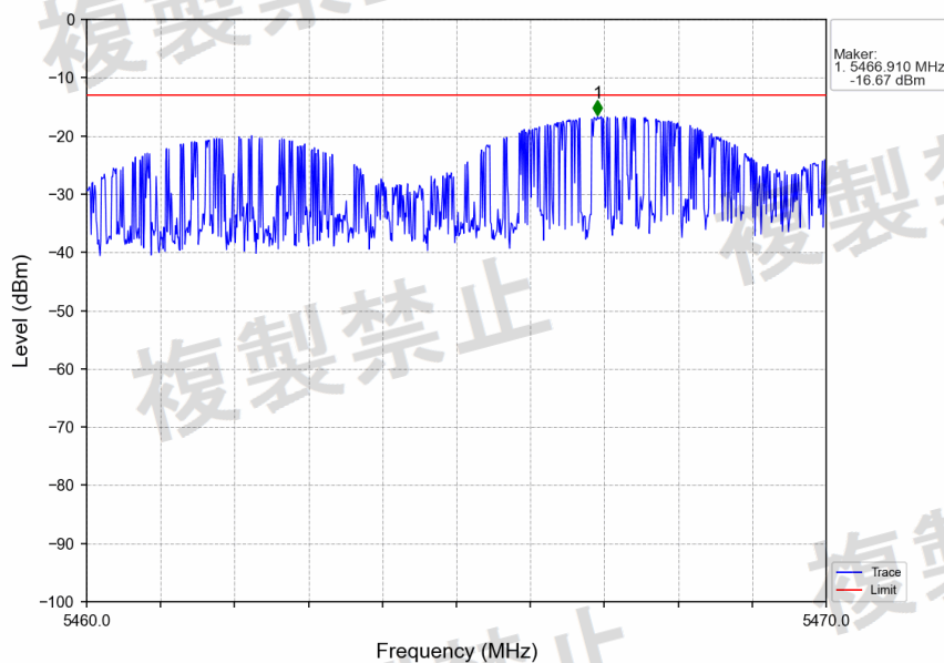
802.11ax(HEW40)_LCH_5510MHz_RU484_Left_Ant2_NTNV
