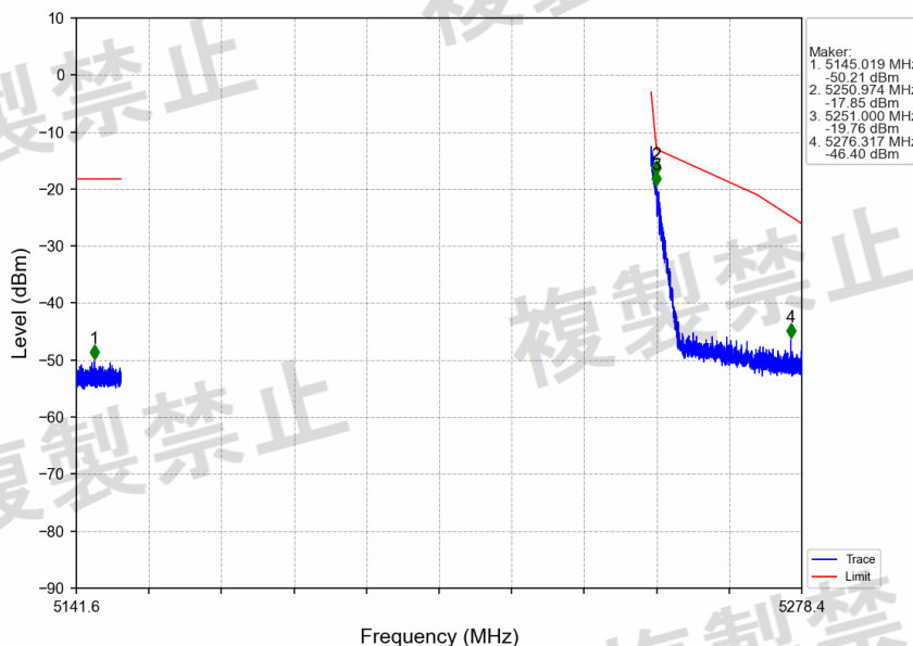
802.11n(HT40)_HCH_5230MHz_Ant2_NTNV
