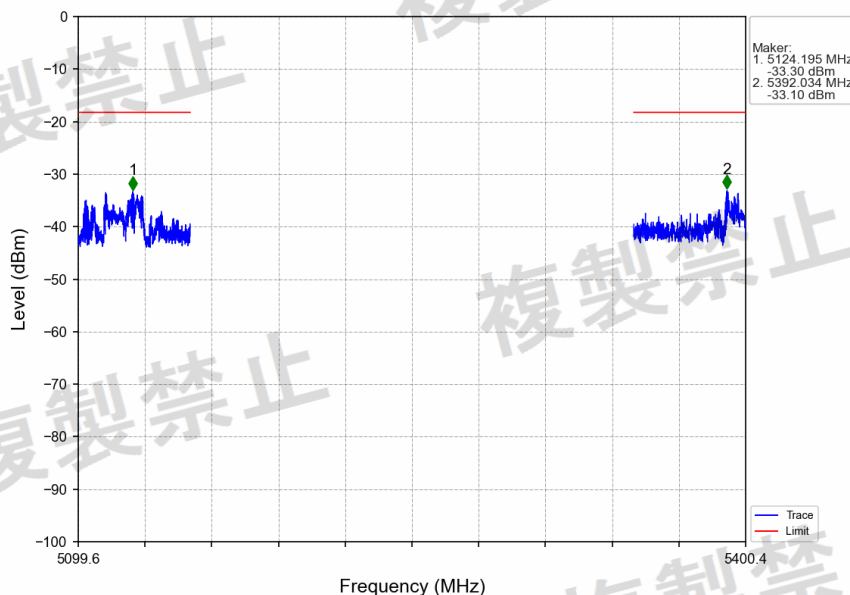
802.11ax(HEW160)_MCH_5250MHz_2xRU996_Left_Ant2_NTNV
