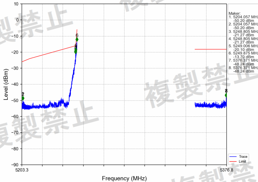
802.11be(EHT80)_MCH_5290MHz_RU996_Left_MIMO_NTNV
