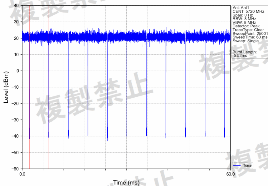
802.11a_HHCH_5720MHz_Ant1_NTNV
