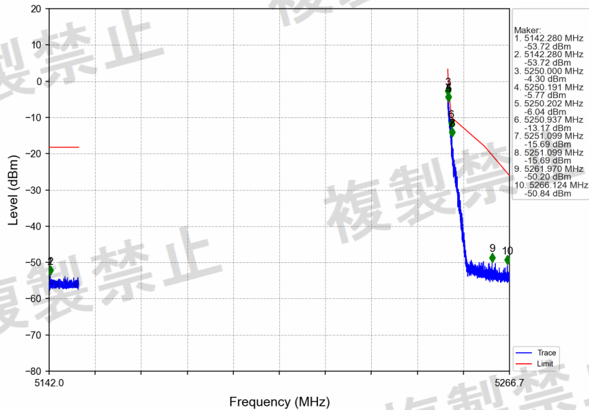
802.11be(EHT20)_HCH_5240MHz_RU242_Left_MIMO_NTNV
