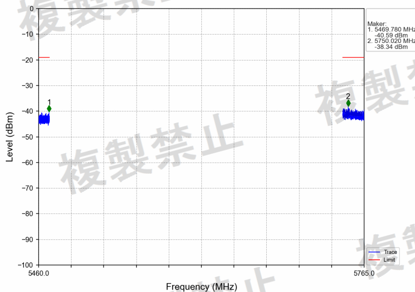
802.11be(EHT20)_HCH_5700MHz_RU242_Left_Ant2_NTNV
