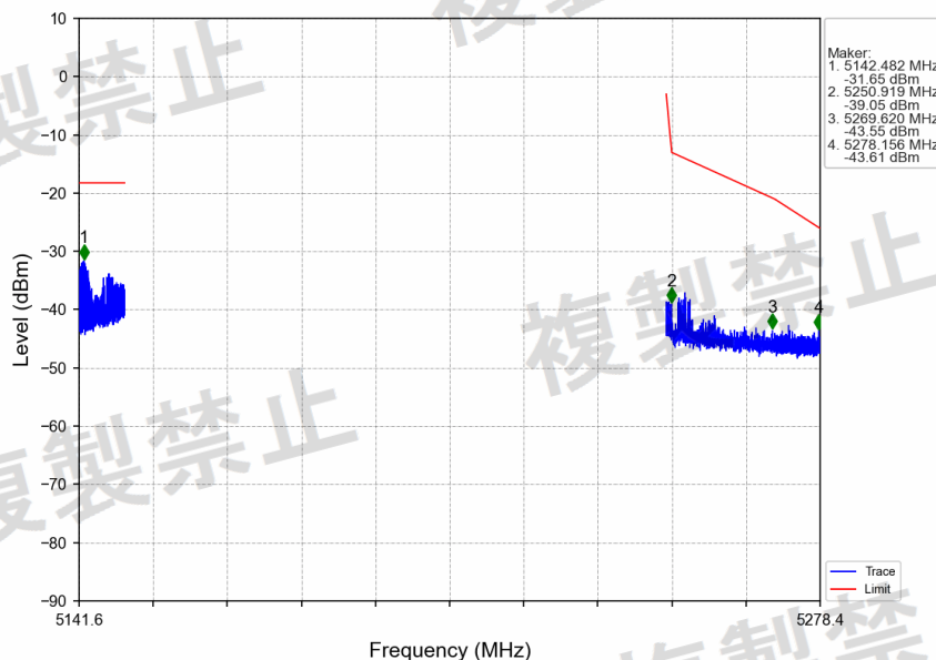
802.11ax(HEW40)_LCH_5190MHz_RU484_Left_Ant2_NTNV
