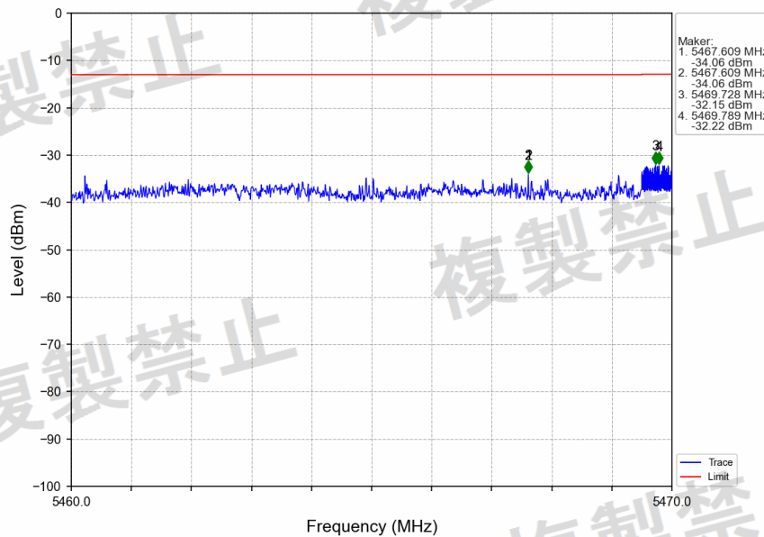
802.11ax(HEW80)_LCH_5530MHz_RU996_Left_MIMO_NTNV
