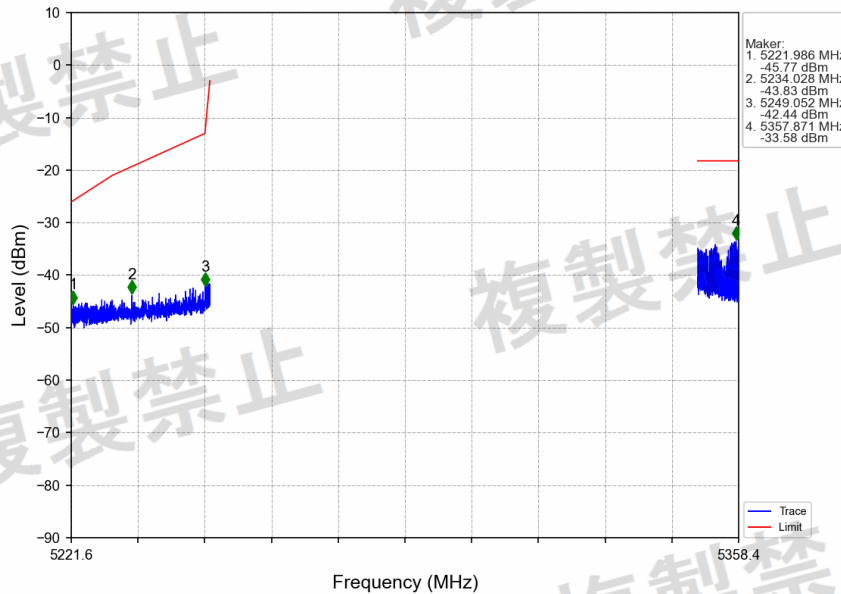
802.11ax(HEW40)_HCH_5310MHz_RU484_Left_Ant2_NTNV
