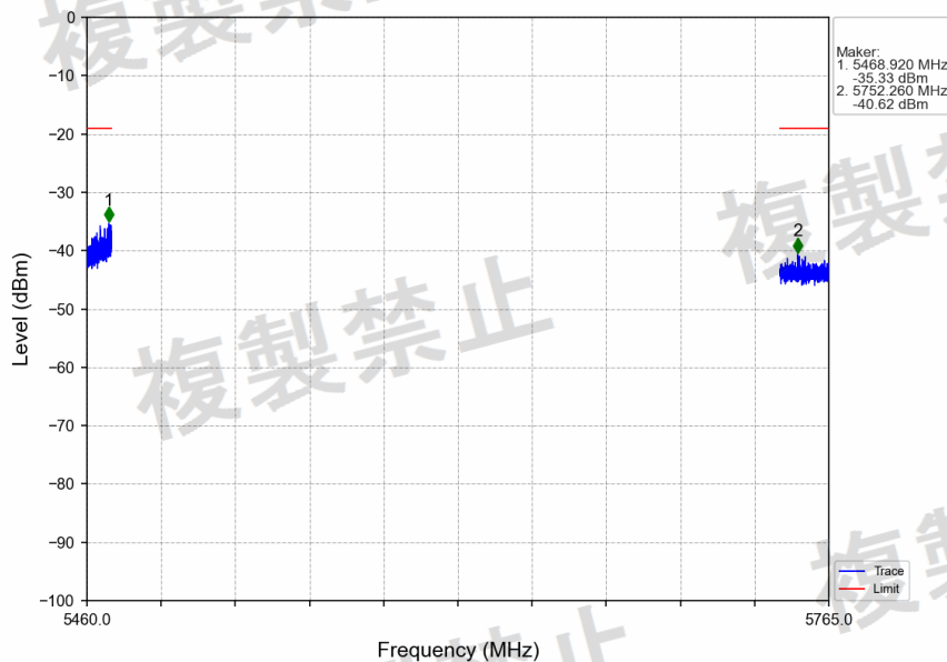
802.11be(EHT20)_LCH_5500MHz_RU242_Left_Ant2_NTNV
