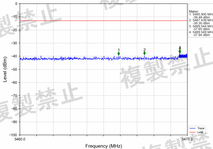
802.11ax(HEW80)_HCH_5610MHz_RU996_Left_MIMO_NTNV
