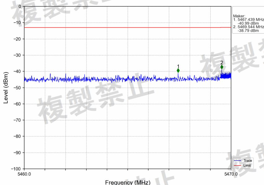
802.11ax(HEW80)_HCH_5610MHz_RU996_Left_Ant2_NTNV
