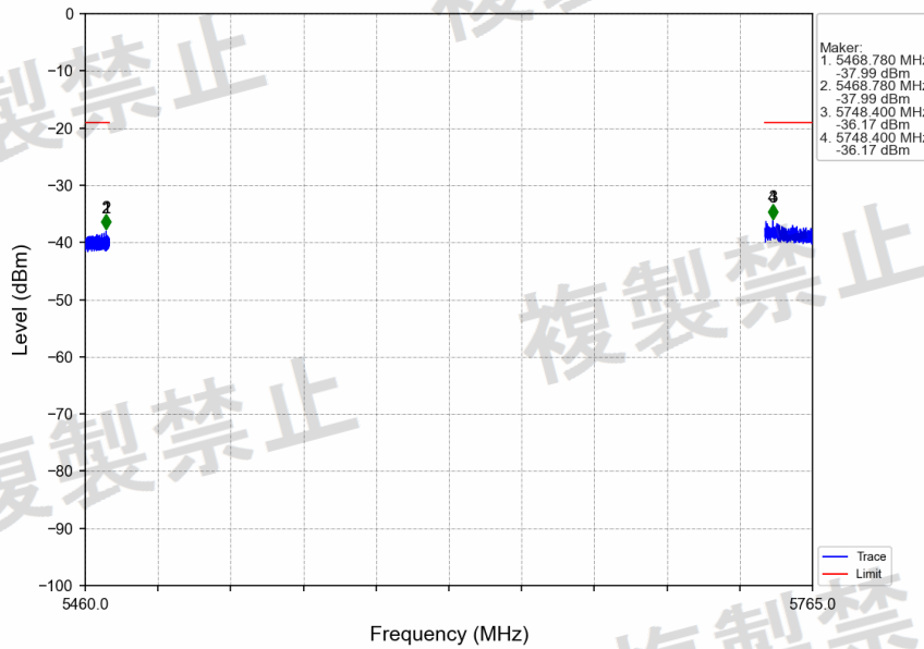
802.11be(EHT20)_HCH_5700MHz_RU242_Left_MIMO_NTNV
