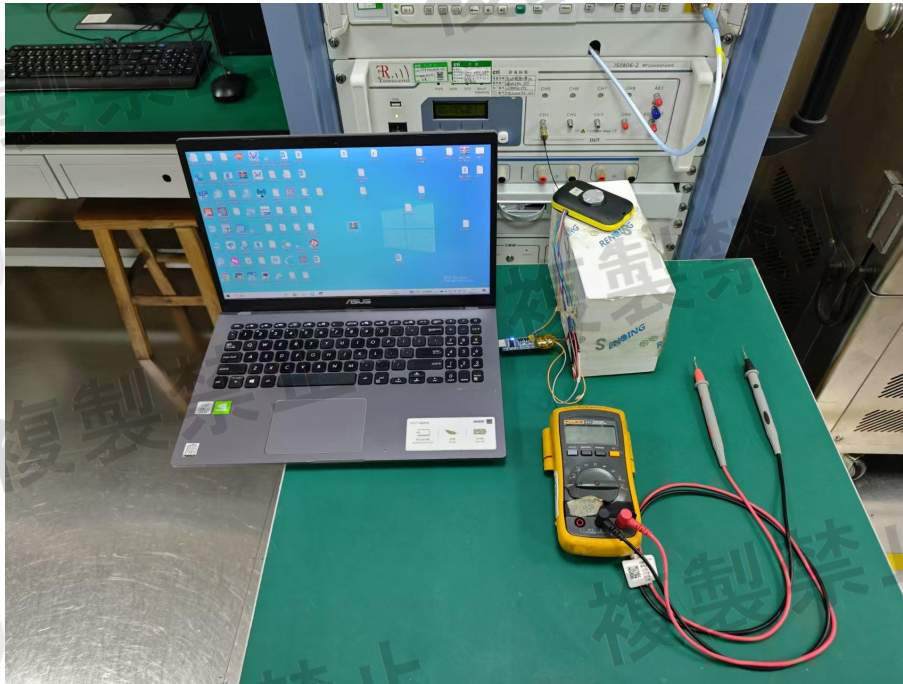
Test Setup-1
