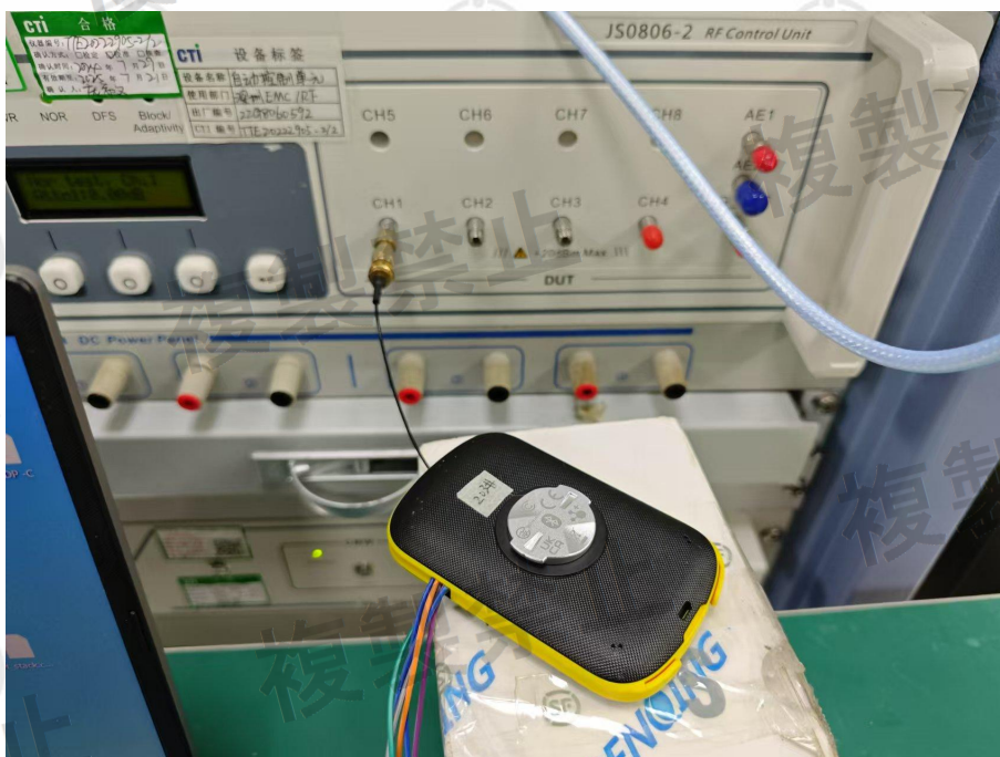
Test Setup-2
