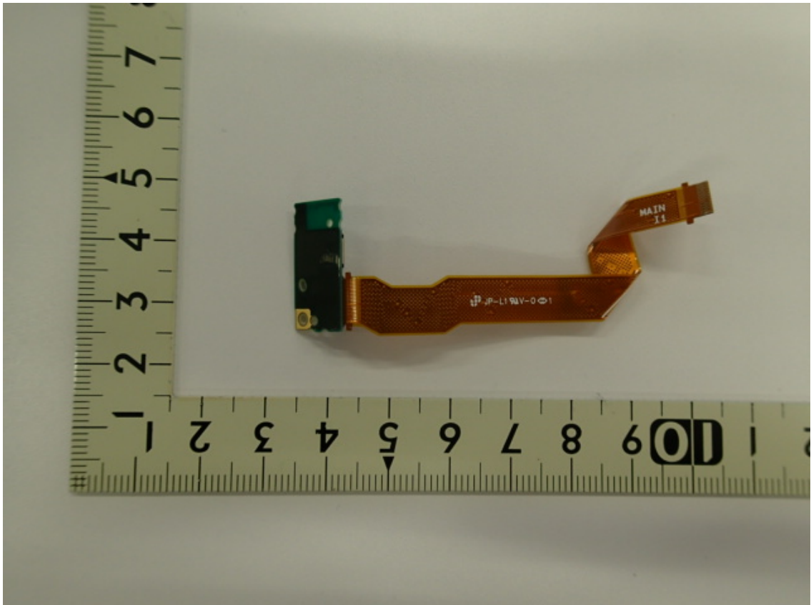
WLAN_BT Module
