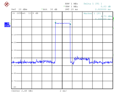
CH78-2DH5
