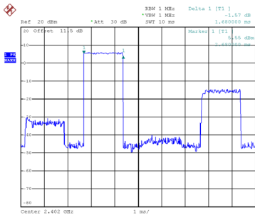
CH00-2DH3
