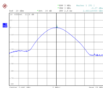
CH39
