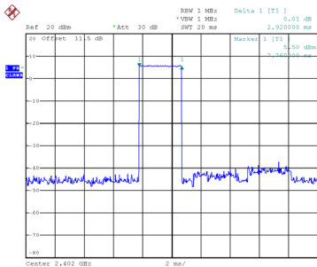
CH00-2DH5
