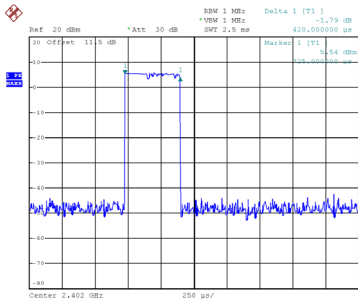
CH00-2DH1
