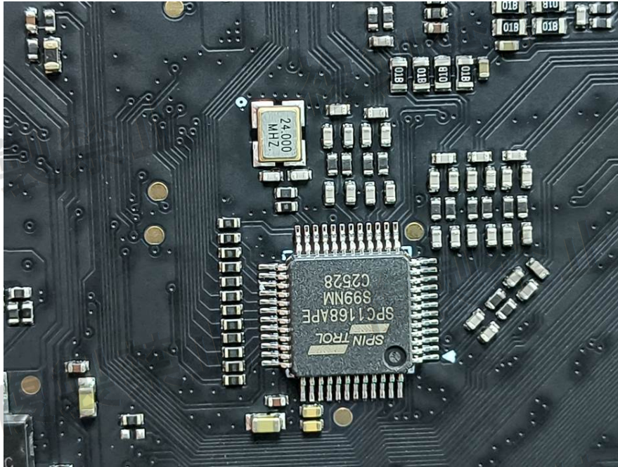
MEGMEET (MPT150-24V-TZ-B)
