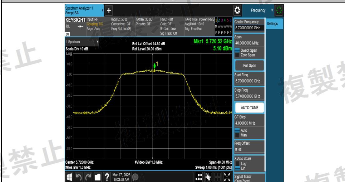
NTNV_11A_Ant1_5720
