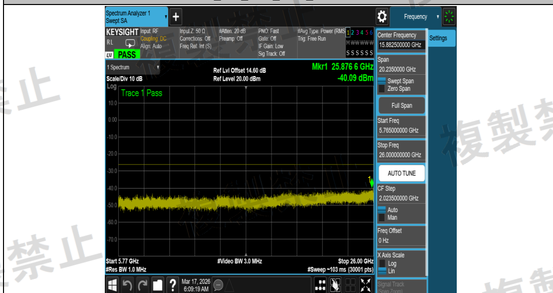
NTNV_11A_Ant1_5720_5765~26000
