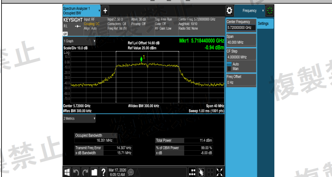
NTNV_11A_Ant1_5720
