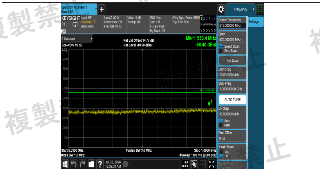
NTNV_11A_Ant1_5580_30~1000
