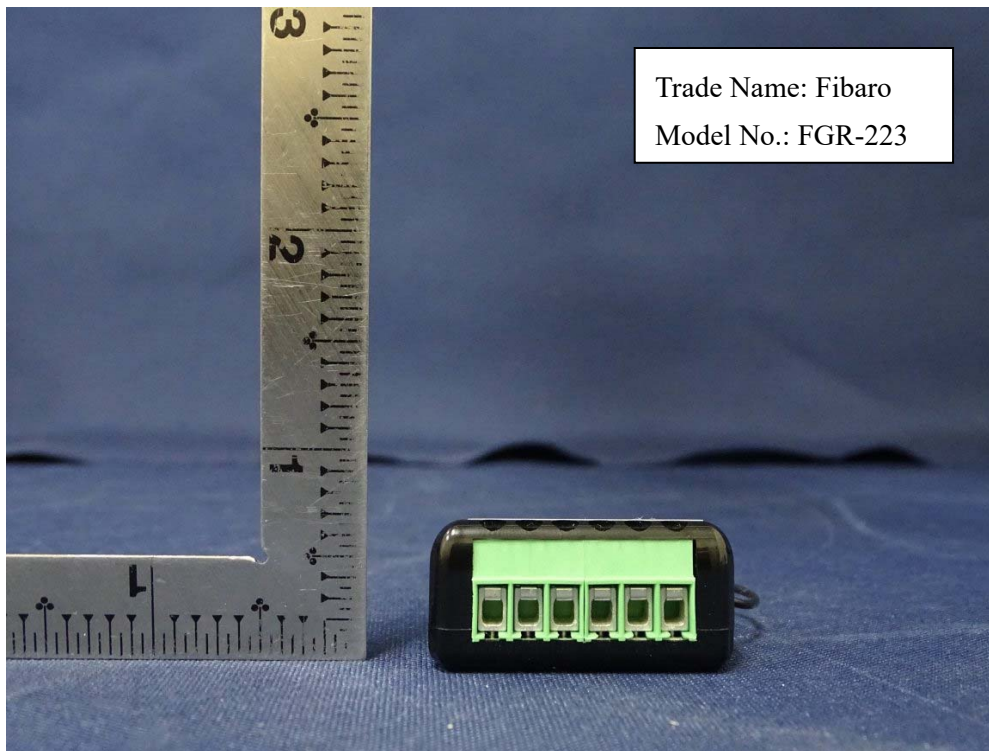
(3) EUT Photo
