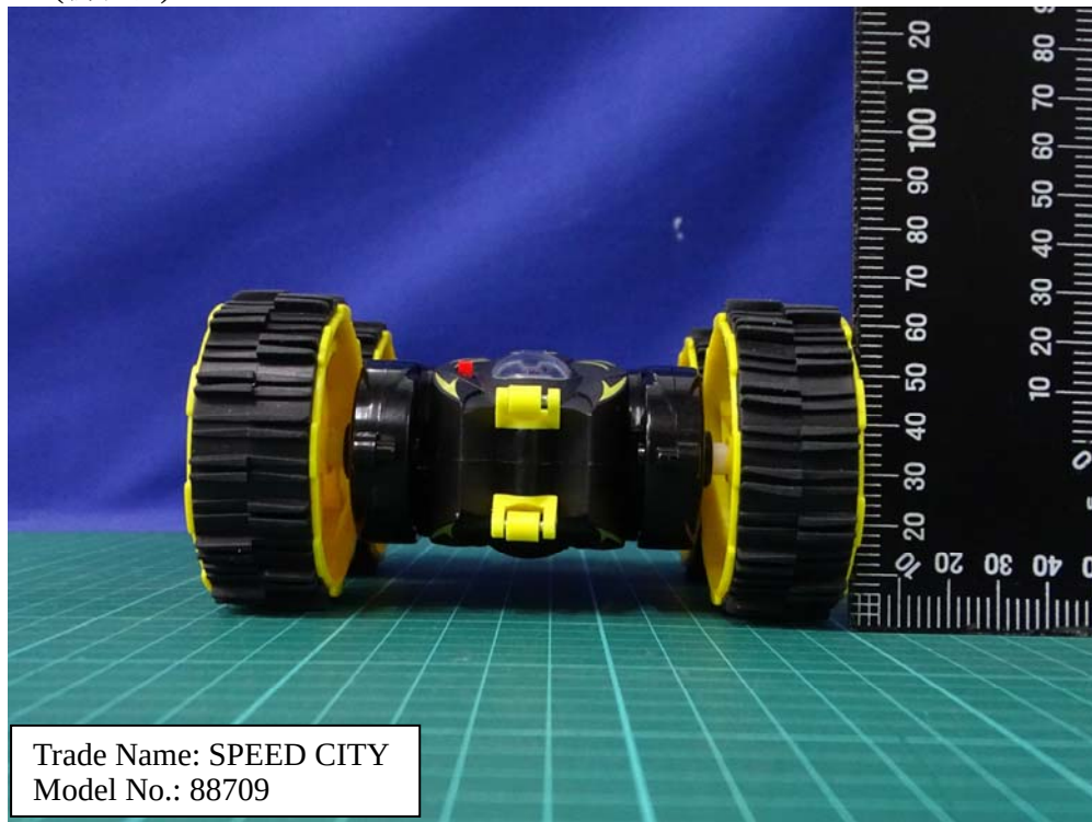
(5) EUT Photo (接收器)
