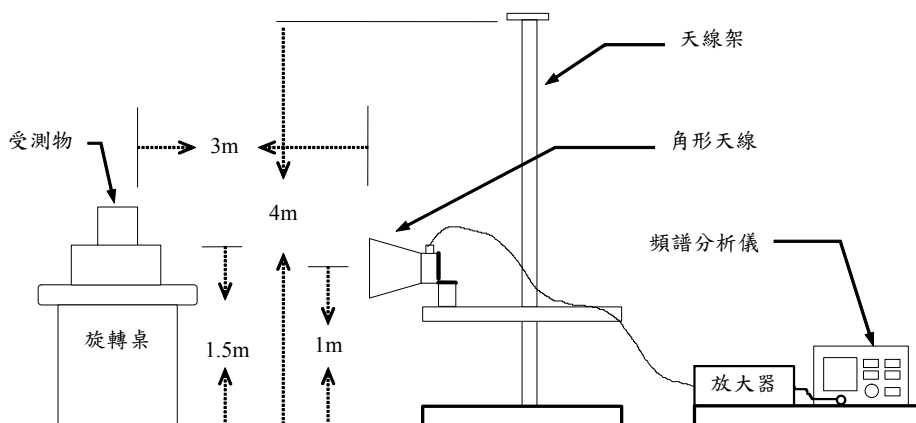
圖 2：量測頻率高於 1GHz 之測試配置
