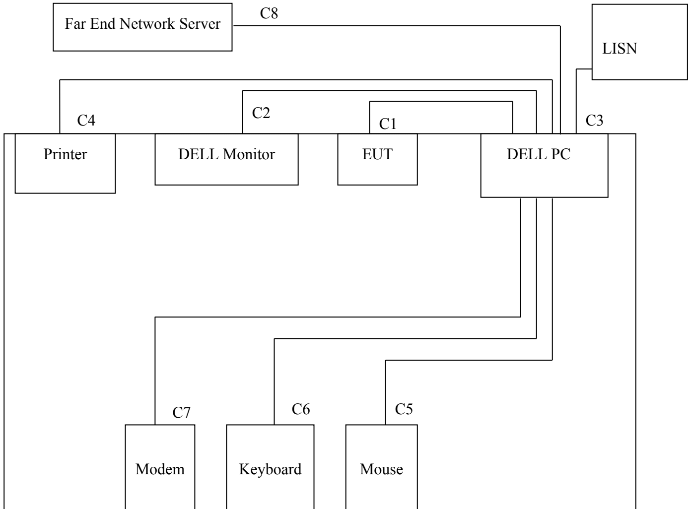
圖(一) 電源傳導測試系統組成示意圖
