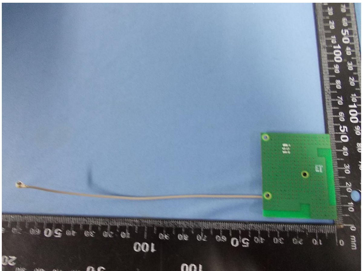
Antenna
