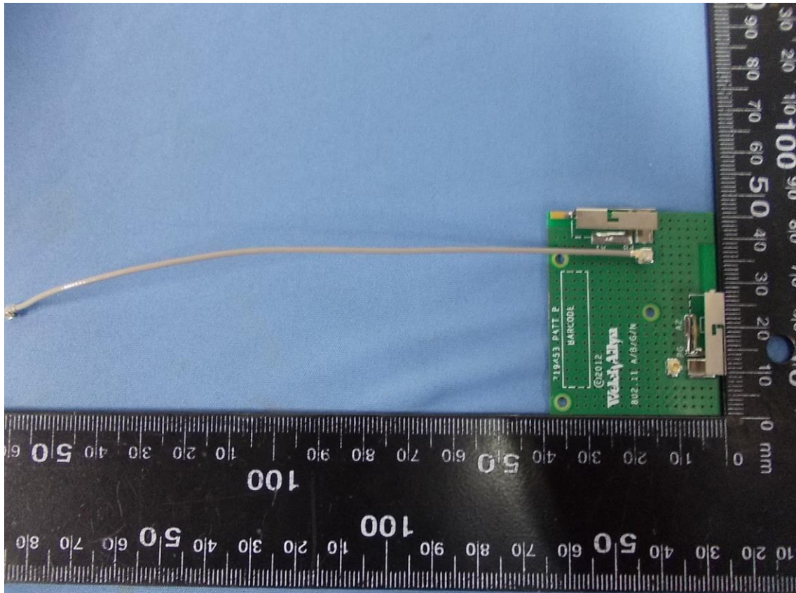
Antenna
