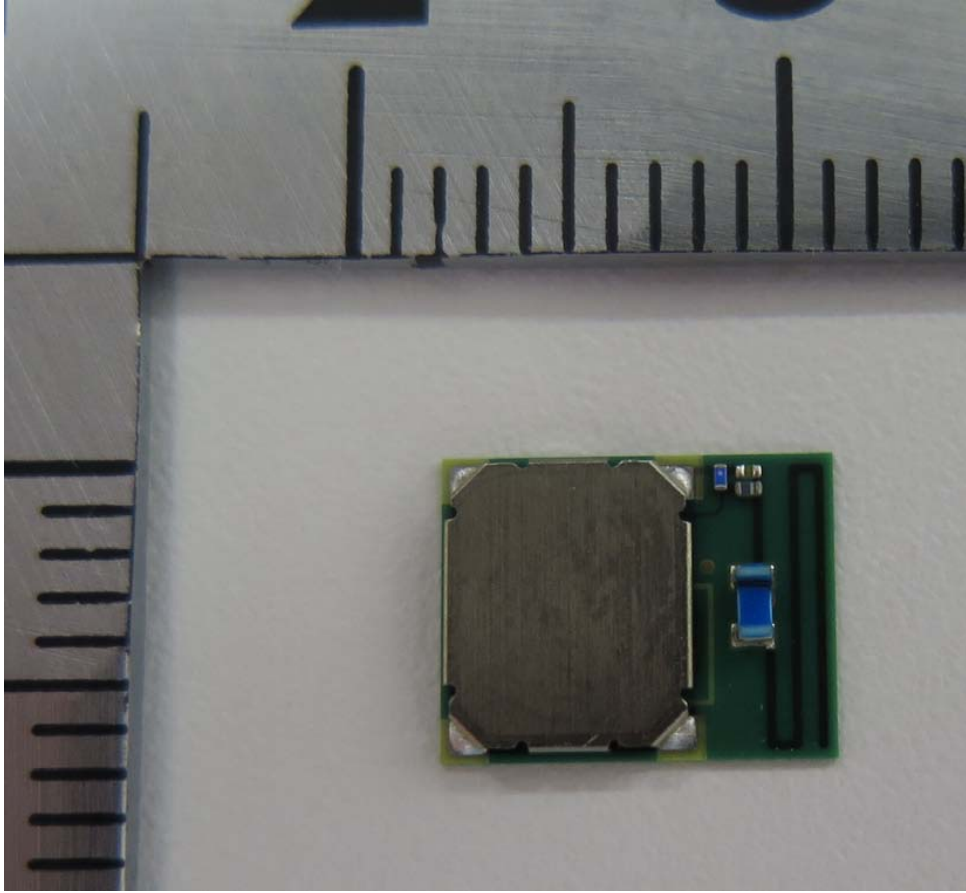
BLE Module (WM500)
