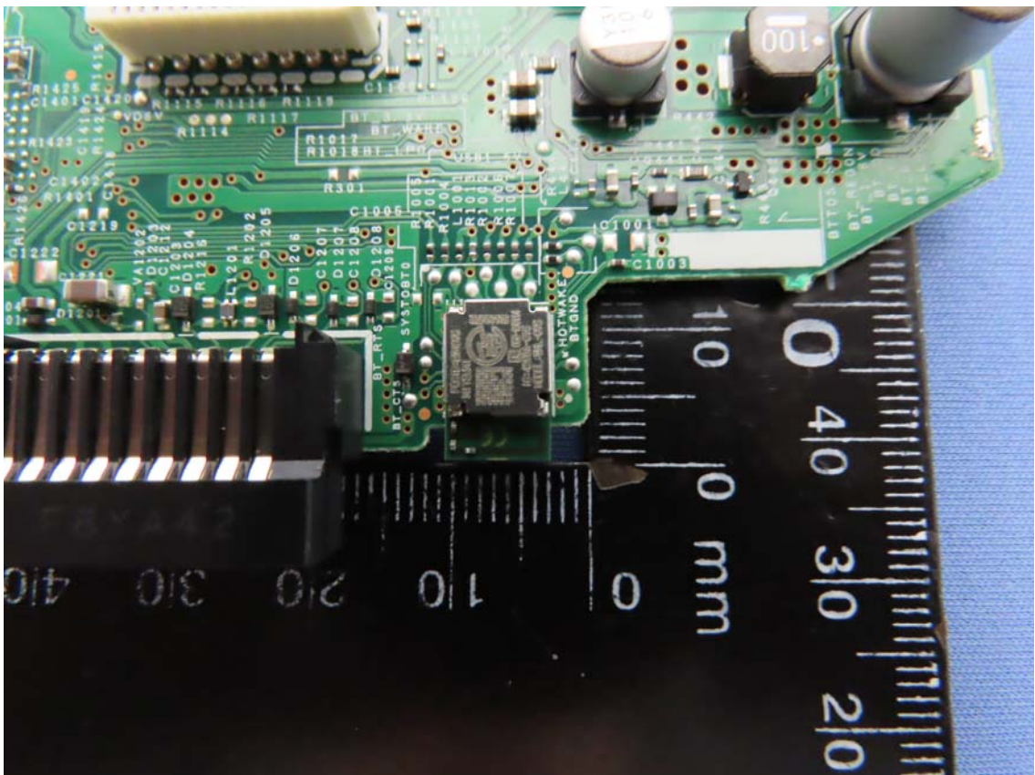
電路板正面照一
