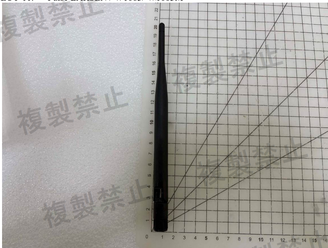
EUT-11. Pulse LARSEN / W1063/ W1063M
