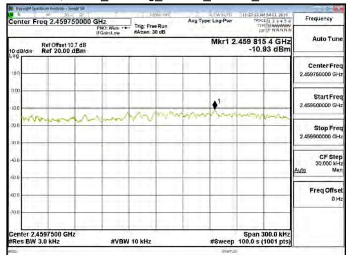
功率密度_802.11g_20MHz_Chain0_2462MHz
