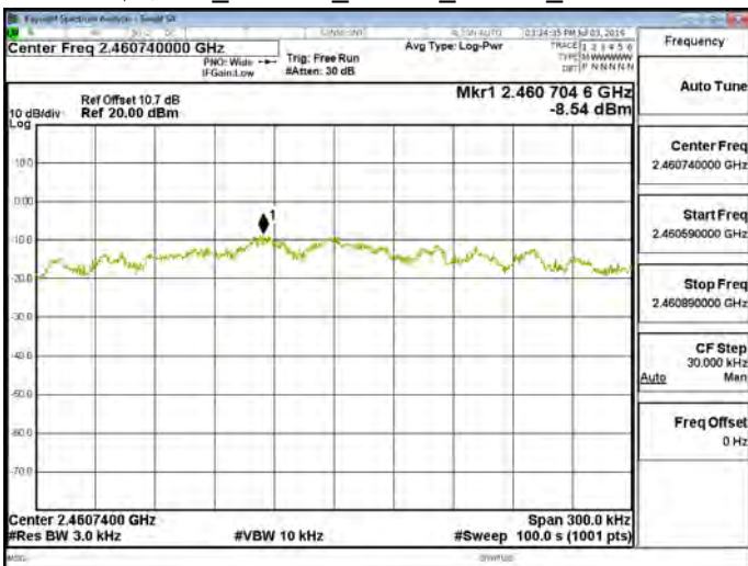
功率密度_802.11n_20MHz_Chain0_2462MHz
