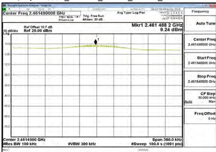
參考限制值_802.11b_20MHz_Chain0_2462MHz
