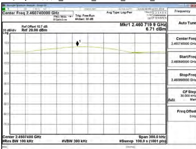
參考限制值_802.11n_20MHz_Chain0_2462MHz
