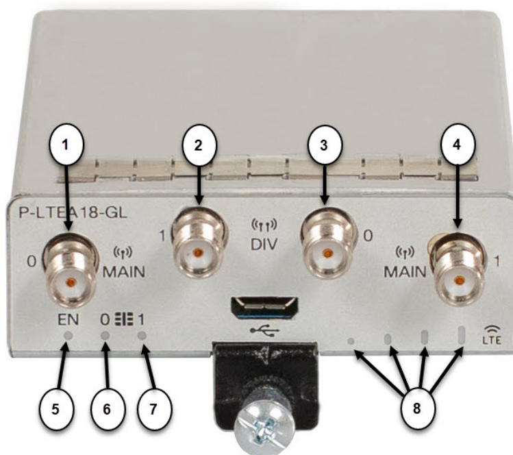
図 3: P-LTEA18-GL プラグブル インターフェイス モジュール
