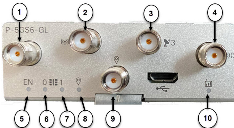
図 4: 5G セルラー プラガブルインターフェイス モジュール
