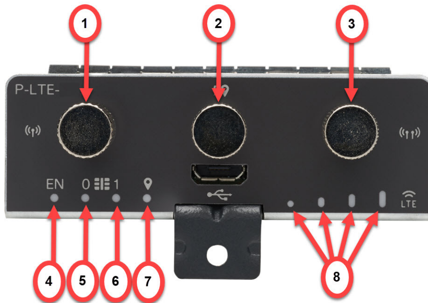
図 2: P-LTE-x プラガブル インターフェイス モジュール
