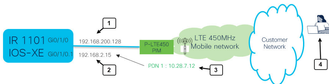
図 11 : P-LTE-450 MHz モジュールトポロジの WebUI の接続
