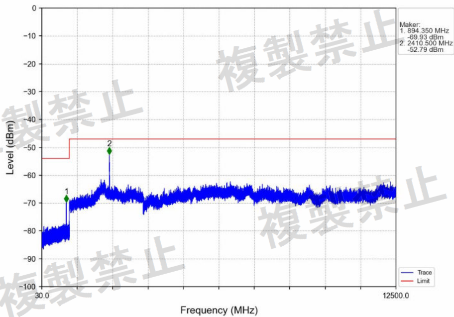
802.11ax(HEW20)_2472MHz_SU_/_Ant1 (SISO)_NTNV
