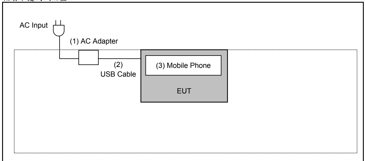
幅射干擾測試配置
