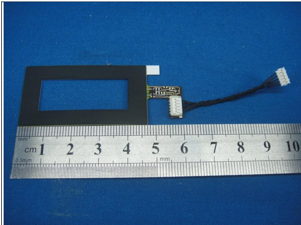
Antenna 8(Brand : SAA / Model : LX7828-12-000-R)
