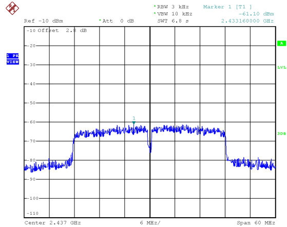
2437 MHz
