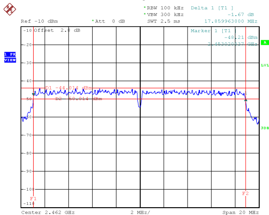
2462 MHz
