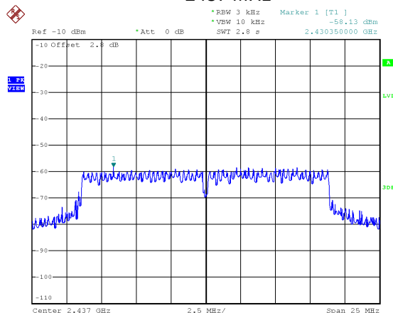
2437 MHz
