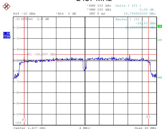
2437 MHz
