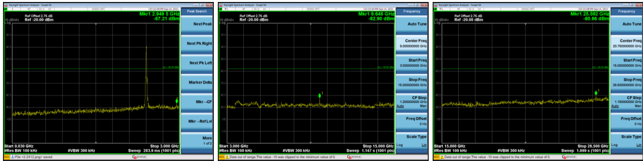
2437 MHz -10 倍諧波
