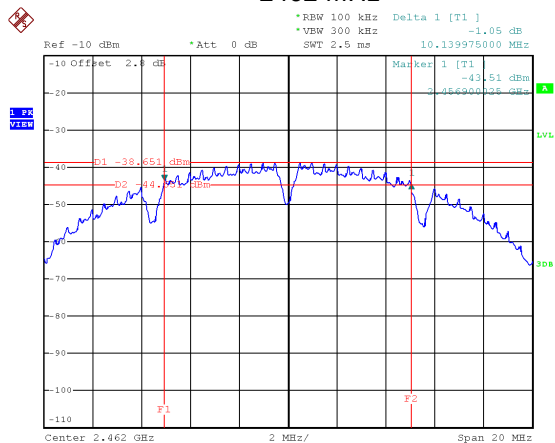
2462 MHz
