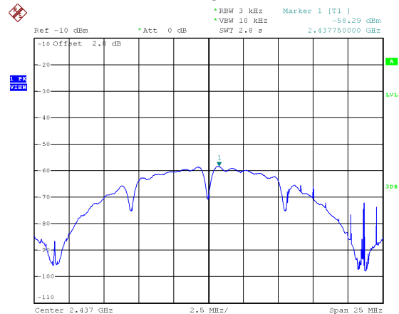
2437 MHz
