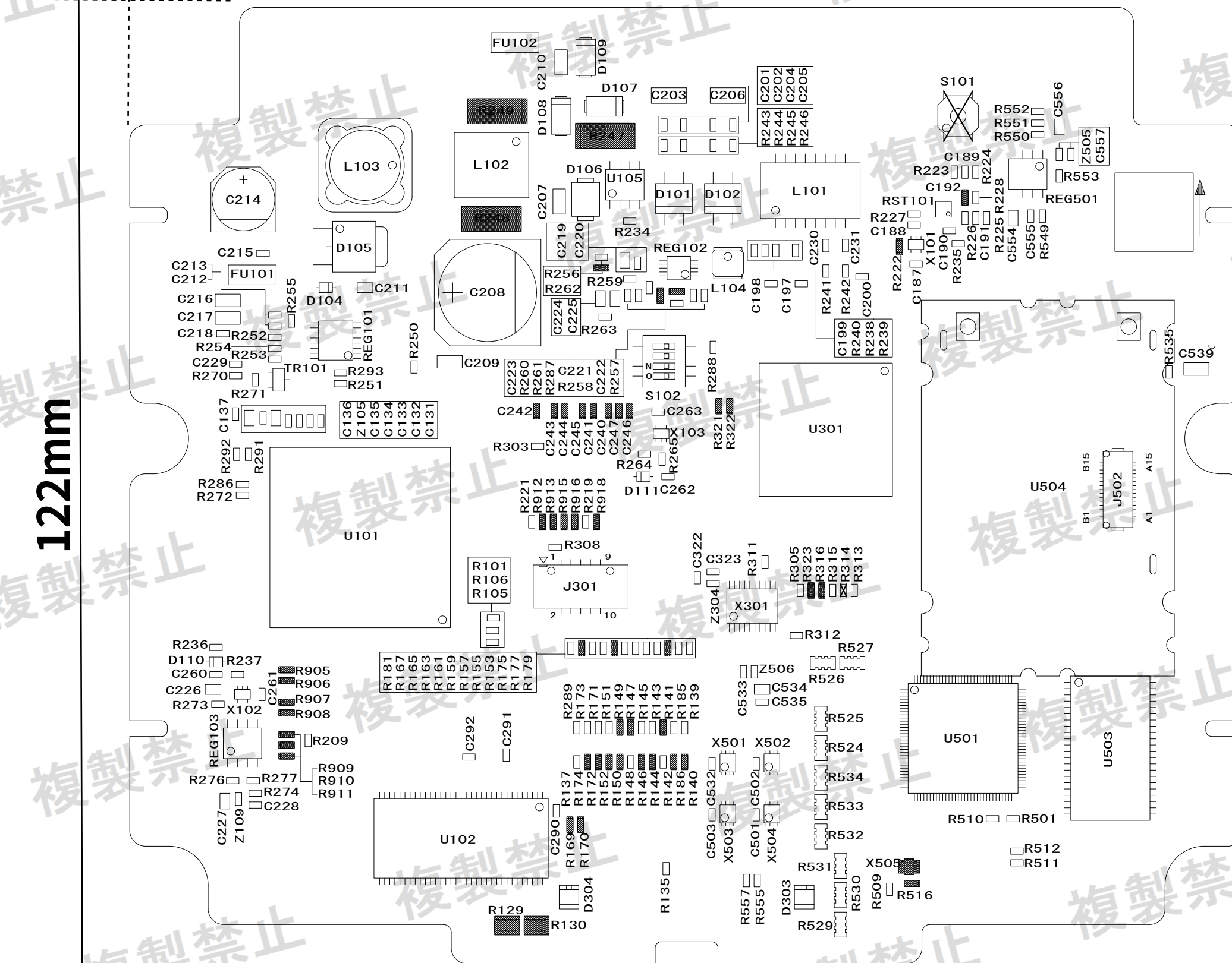
【部品配置図】 BS401 (部品面)
