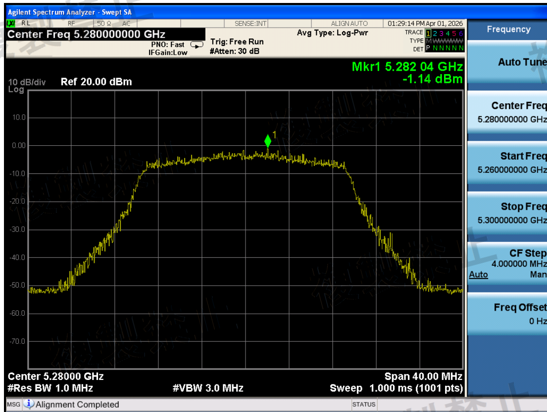
W53\Antenna Power Error\802.11ax HE20\1-5280-TX0-N
