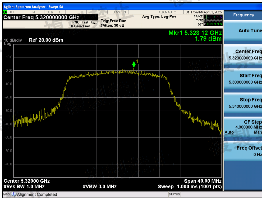
W53\Antenna Power Error\802.11ax HE20\1-5320-TX1-N
