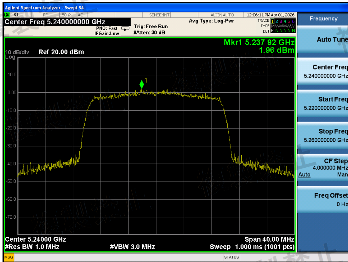
W52\Antenna Power Error\802.11ax HE20\1-5240-TX0-N
