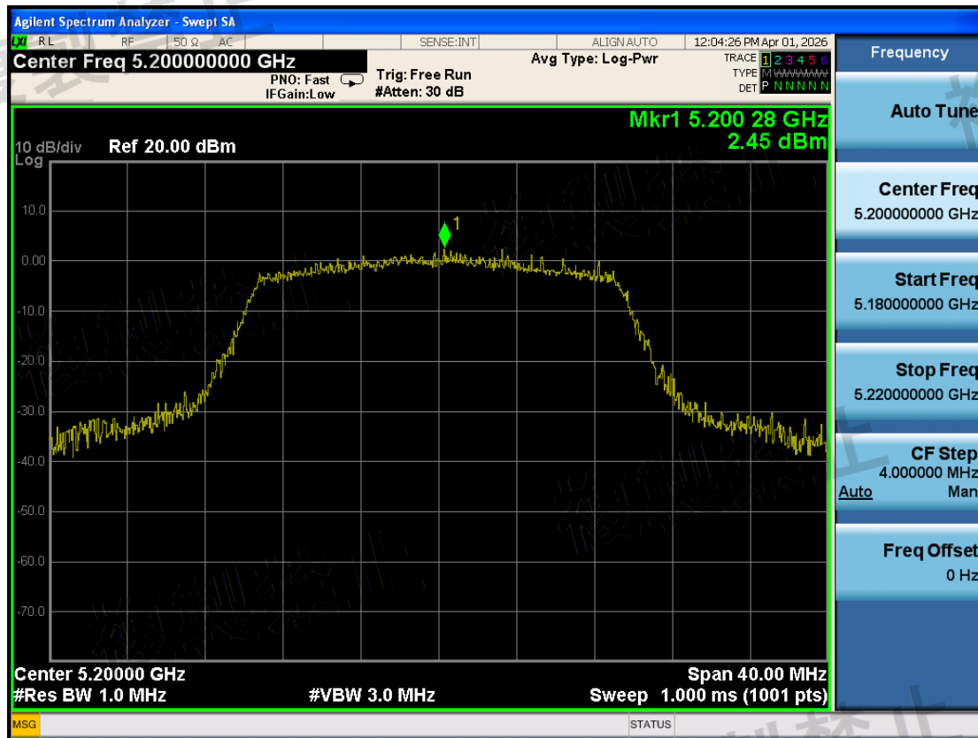
W52\Antenna Power Error\802.11ax HE20\1-5200-TX0-N
