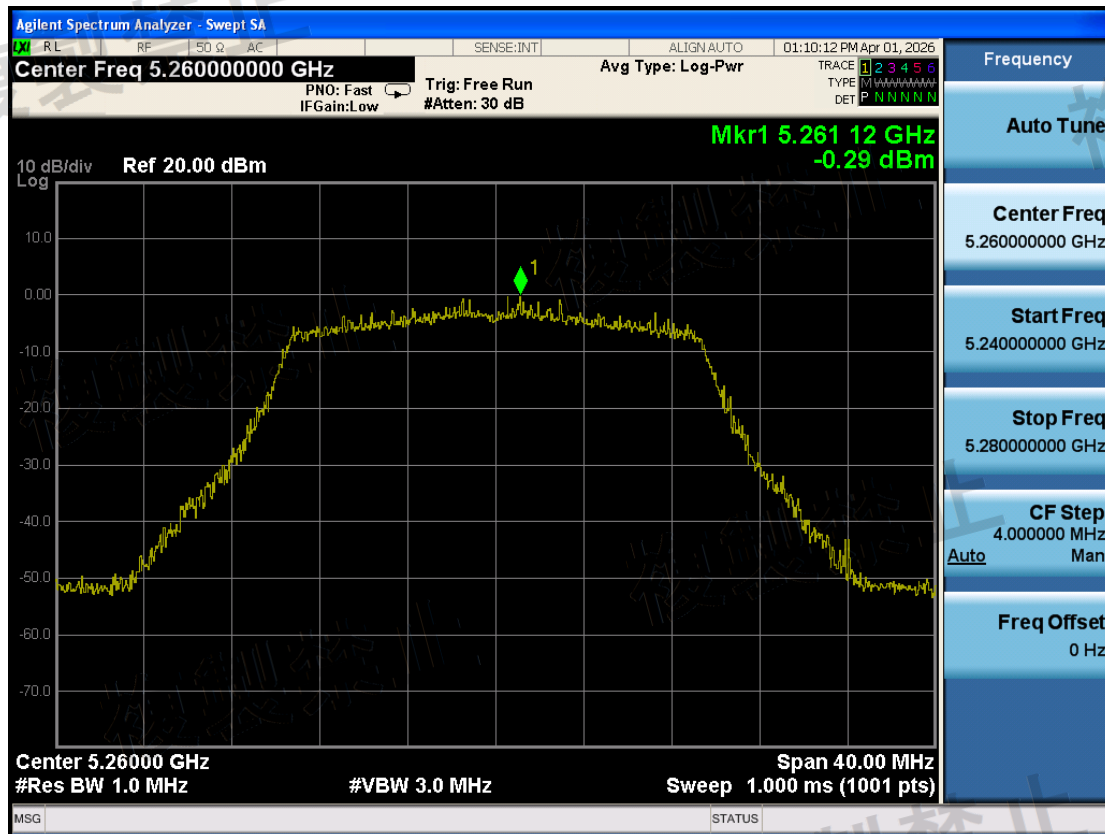
W53\Antenna Power Error\802.11ax HE20\1-5260-TX0-N
