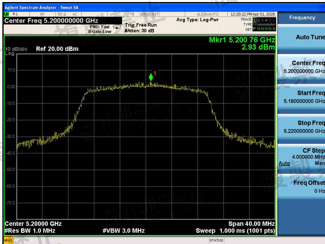
W52\Antenna Power Error\802.11ax HE20\1-5200-TX1-N
