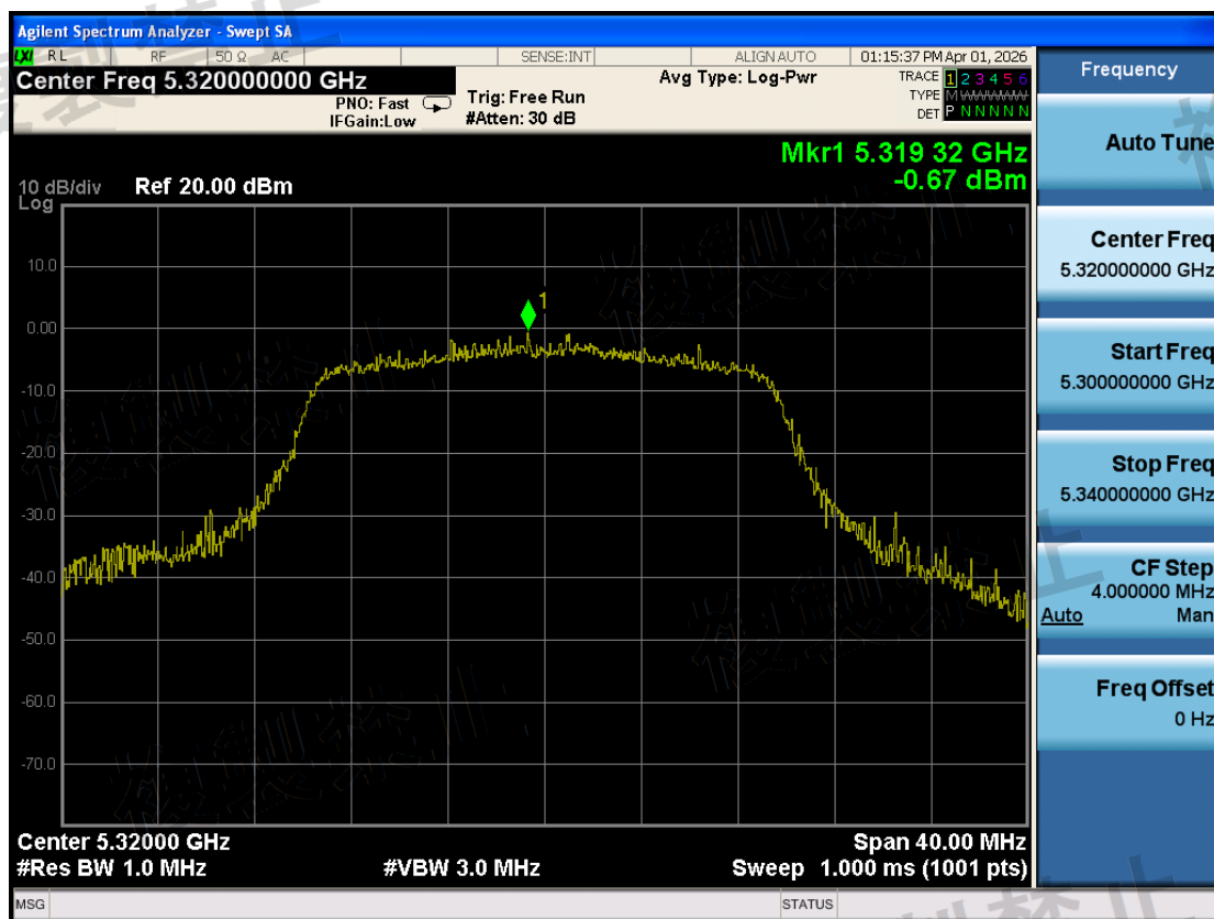
W53\Antenna Power Error\802.11ax HE20\1-5320-TX0-N
