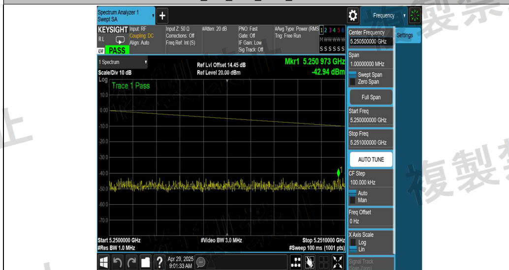
NTNV_11A_Ant1_5220_5250~5251
