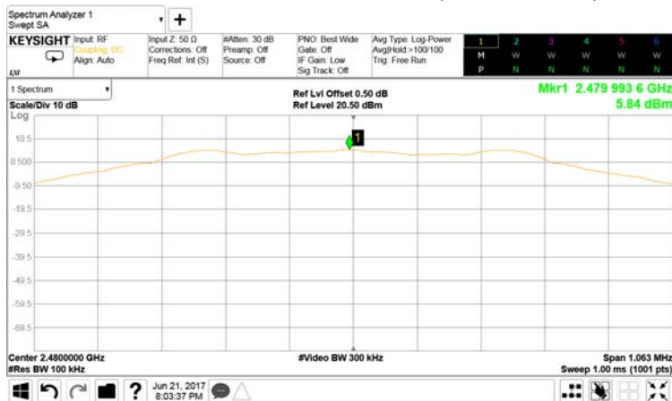
圖三. 功率密度，頻率: 2480MHz (BLE, GFSK)
