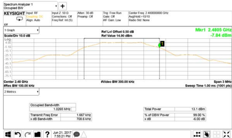
圖三. 6dB 頻寬，頻率: 2480MHz (BLE, GFSK)
