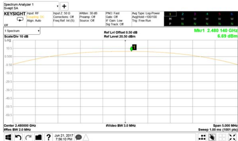
圖三. 峰值輸出功率，頻率: 2480MHz (BLE, GFSK)
