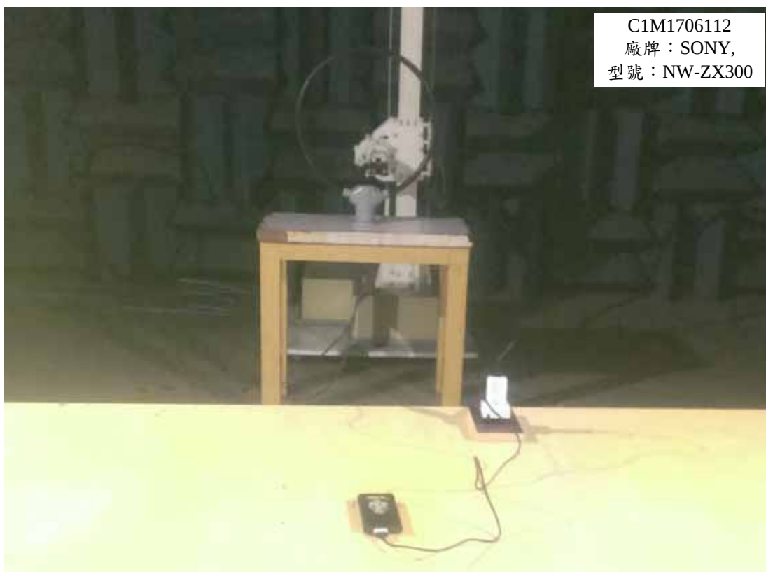
平放(電源供應器電池供電)
