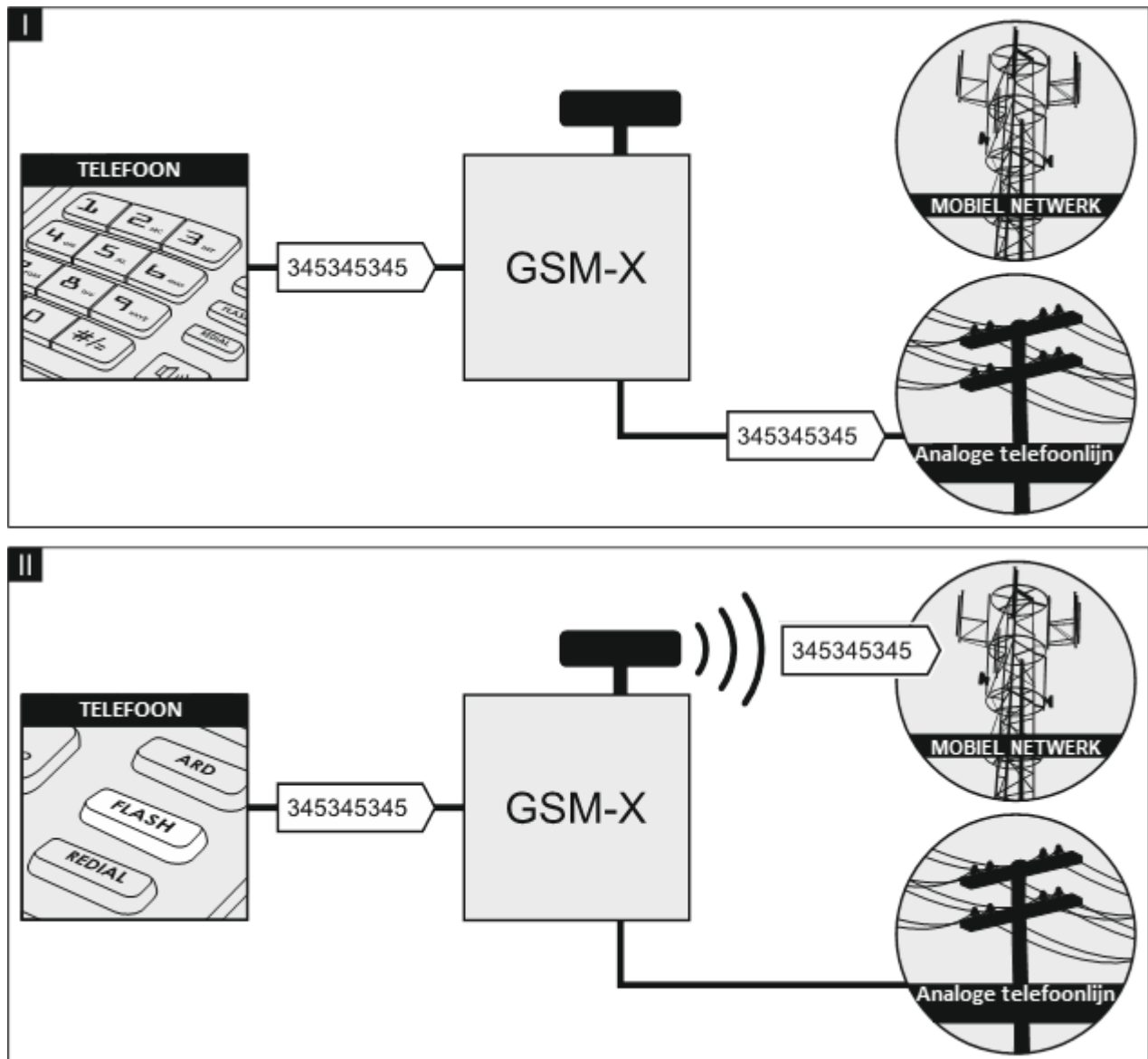
Afb. 38. Schakelen tussen de primaire en back-up communicatie kanalen met de FLASH toets.
