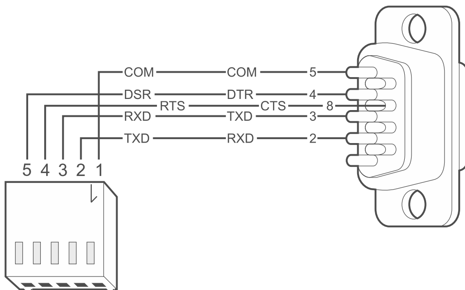
Afb. 16. De RS-232 poorten op de module en computer aansluiten. Getoond aan de linkerzijde is de PIN-5 stekker. Getoond aan de rechterzijde is de DB-9 female stekker (aanzicht soldeerzijde).
