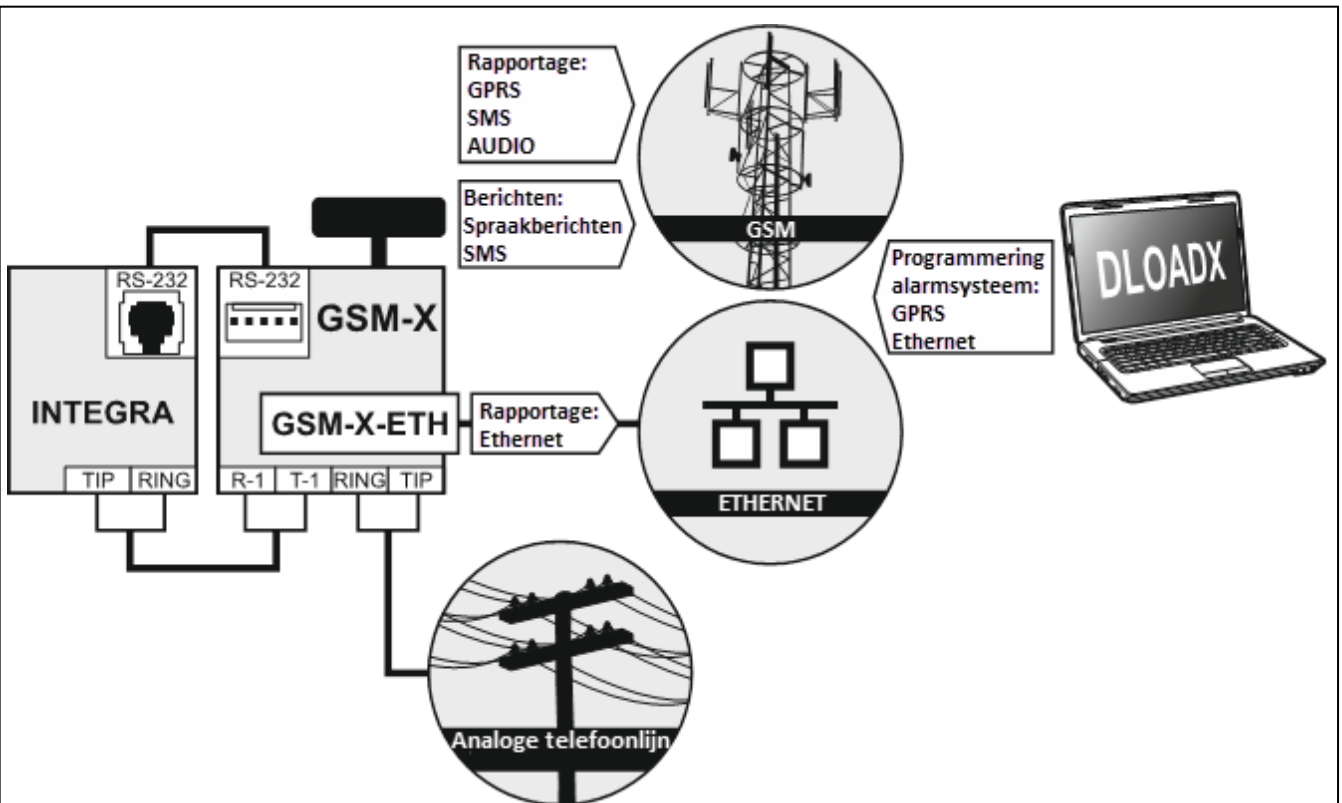
Afb. 6. Module samenwerkend met het INTEGRA / INTEGRA Plus alarmsysteem (de GSM-X-ETH module is geïnstalleerd).
