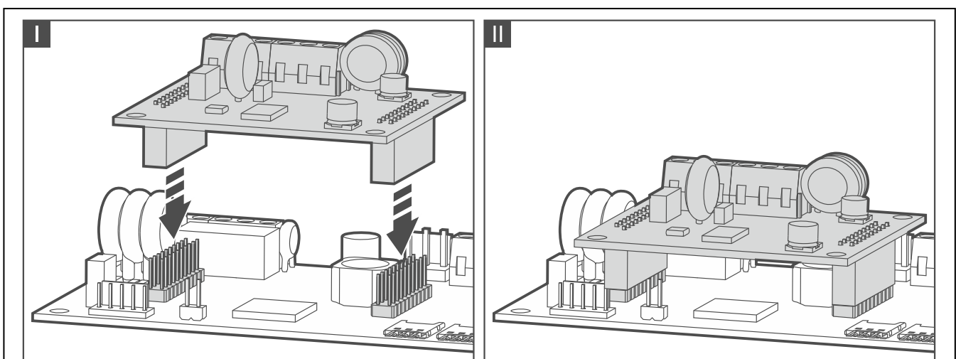
Afb. 21. Plaatsing van de GSM-X-PSTN module op print van de GSM-X module.
