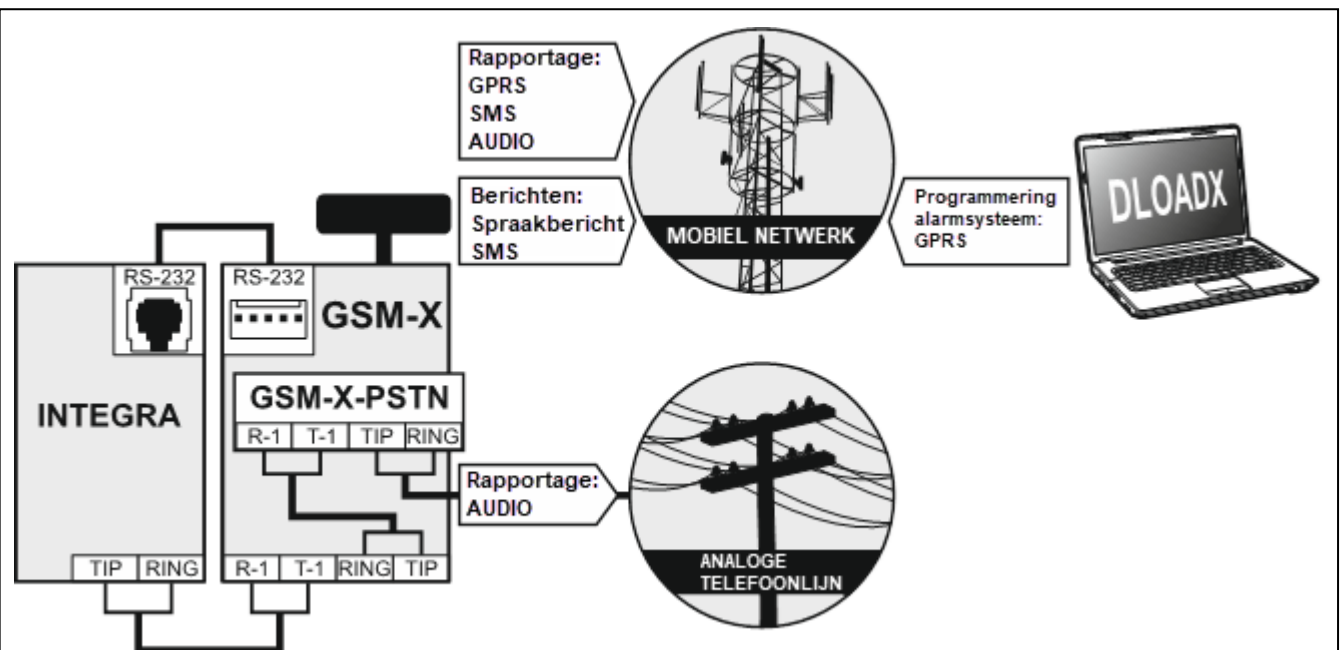
Afb. 7. Module samenwerkend met het INTEGRA / INTEGRA Plus alarmsysteem (de GSM-X-PSTN module is geïnstalleerd).
