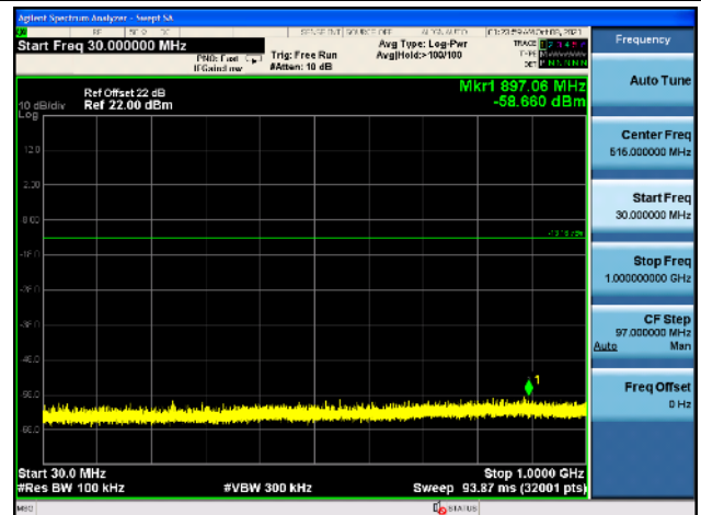
802.11 b CH01 (2412MHz) Ant 0
