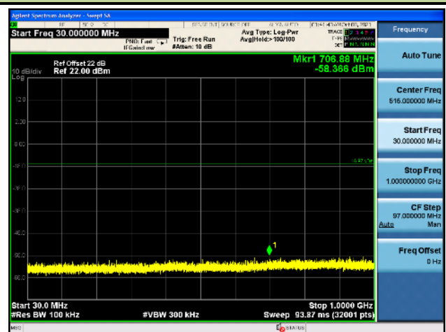
802.11 g CH11 (2462MHz) Ant 1
