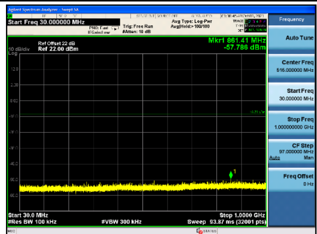
802.11 b CH06 (2437MHz) Ant 1
