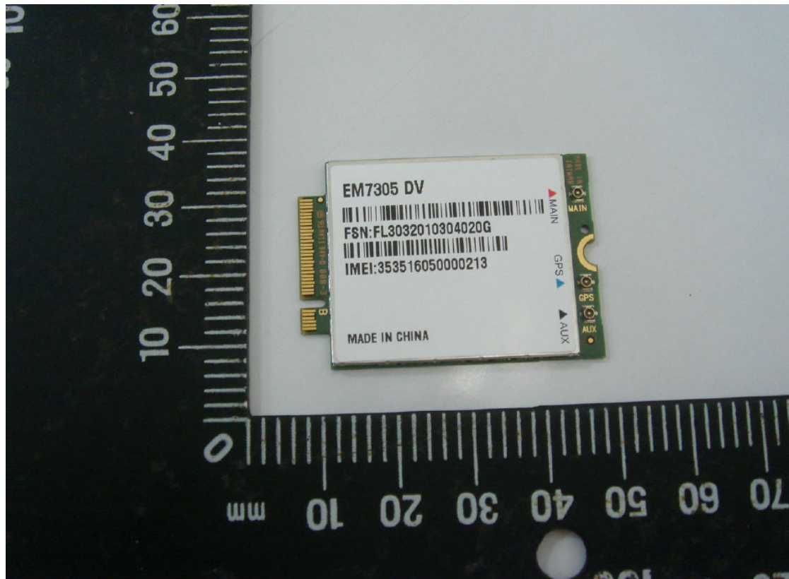
照片一:AirPrime EM7305 正面
