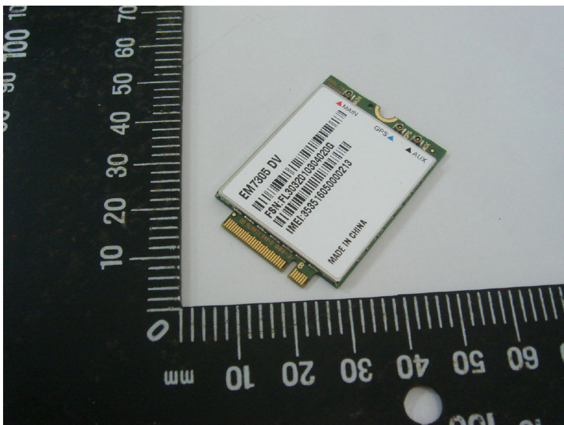
照片三:AirPrime EM7305 側面
