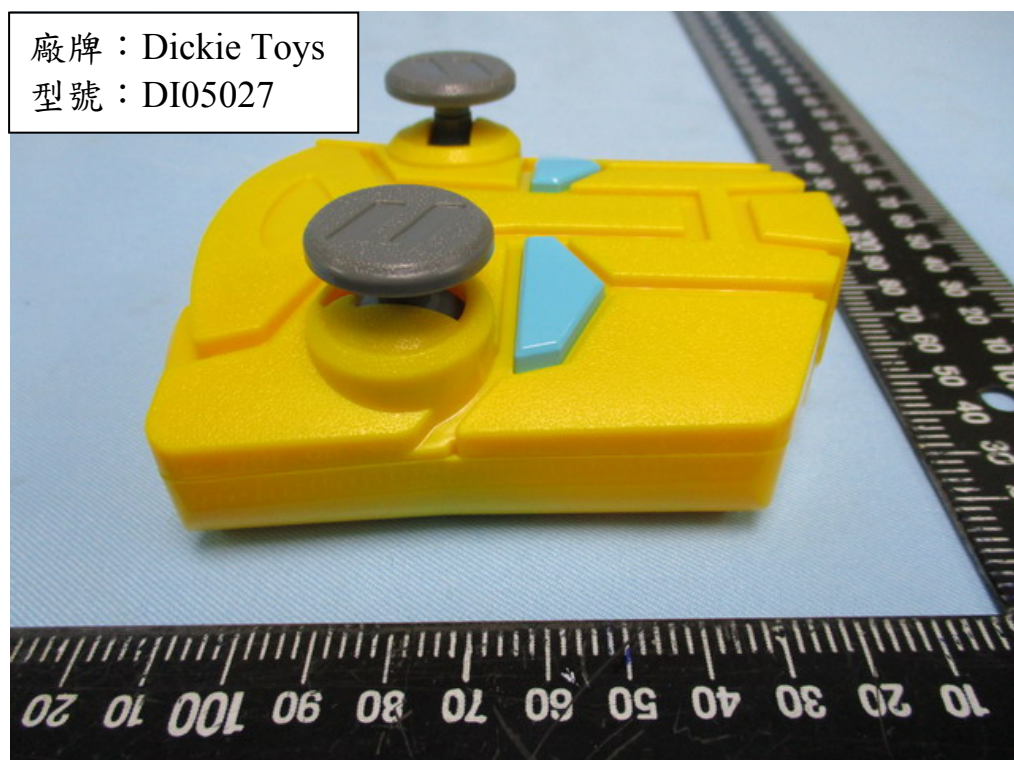
發射機外觀照
