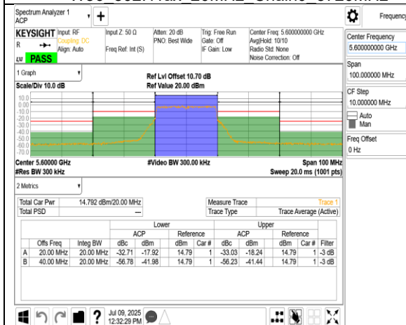
W56 802.11ax 20MHz Chain1 5600MHz
