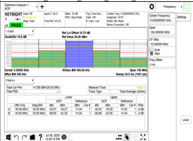
W56 802.11ax 20MHz Chain1 5500MHz
