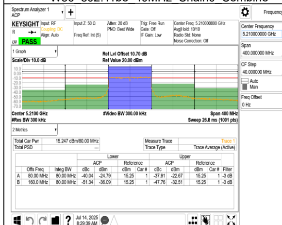
W52 802.11be 80MHz Chain1 5210MHz
