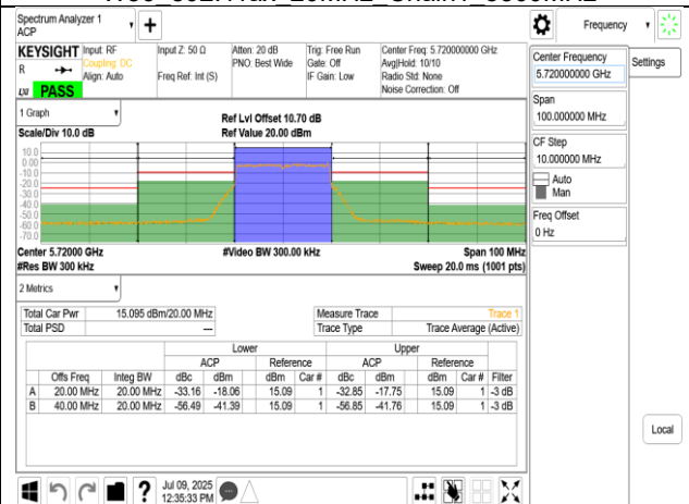
W56 802.11ax 20MHz Chain1 5720MHz
