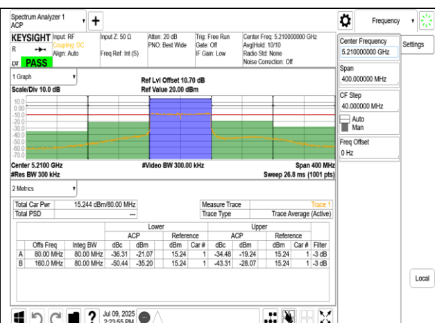
W52 802.11ax 80MHz Chain1 5210MHz
