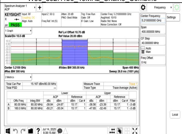
W52 802.11be 80MHz Chain0 5210MHz
