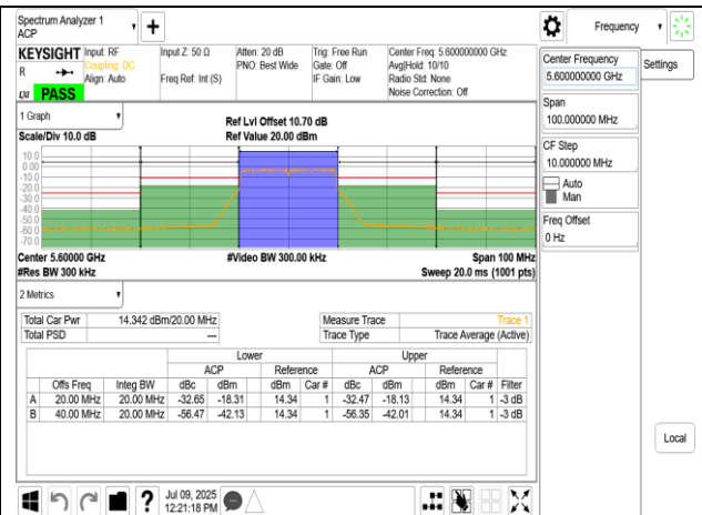
W56 802.11ax 20MHz Chain0 5600MHz
