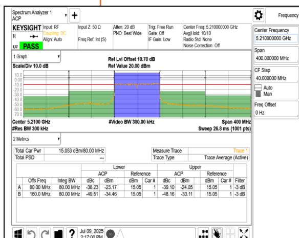
W52 802.11ax 80MHz Chain0 5210MHz
