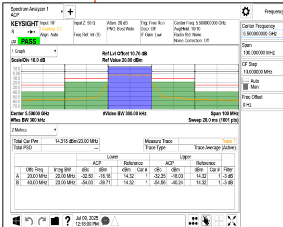
W56 802.11ax 20MHz Chain0 5500MHz
