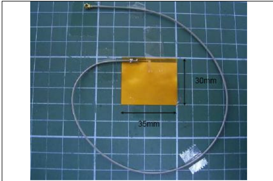
Antenna 13: Brand : Hitachi Cable / Model : HCT01 (Main) / HCT01 (Aux) (For WLAN & BT Used)
