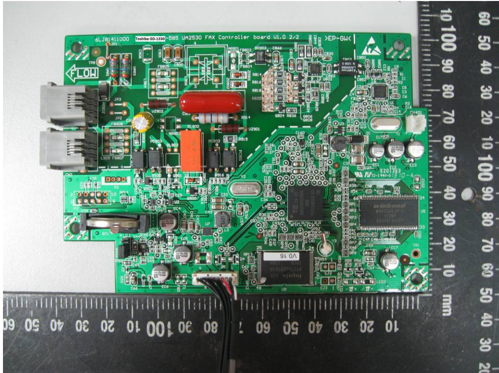
圖 2 傳真卡銅軌面(適用機種數位式複合機廠牌:TOSHIBA;型號: e-STUDIO2507(DP-2507) , e-STUDIO2307(DP-2307) , e-STUDIO2007(DP-2007))
