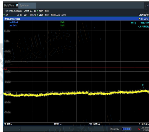
NTVN-11AC40SISO-Ant2-5230-30~5141.6-PAS
