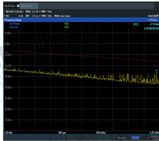
NTNV-11AC80SISO-Ant2-5210-5250~5251-PAS
