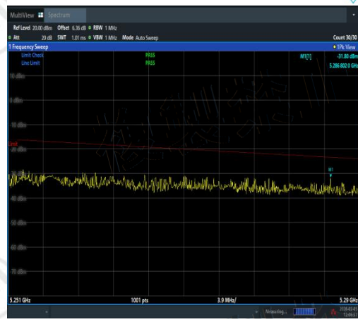
NTNV-11AC80SISO-Ant1-5210-5251~5290-PAS
