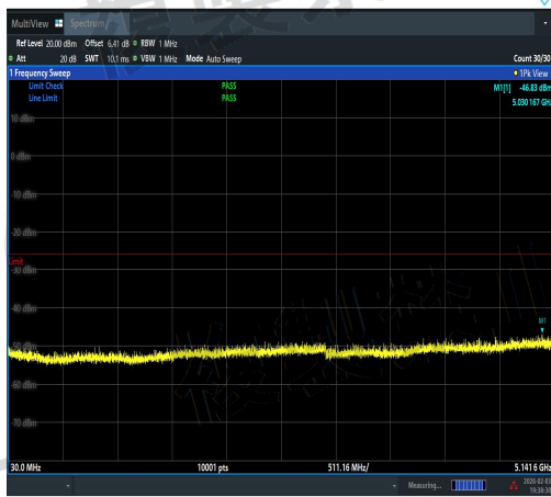
NTVN-11AC40SISO-Ant3-5230-30~5141.6-PAS
