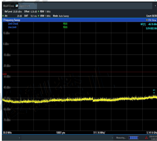
NTVN-11AC40SISO-Ant1-5230-30~5141.6-PAS
