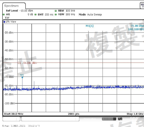
NTVN-11B-Ant1-2472-30~1000-PASS
