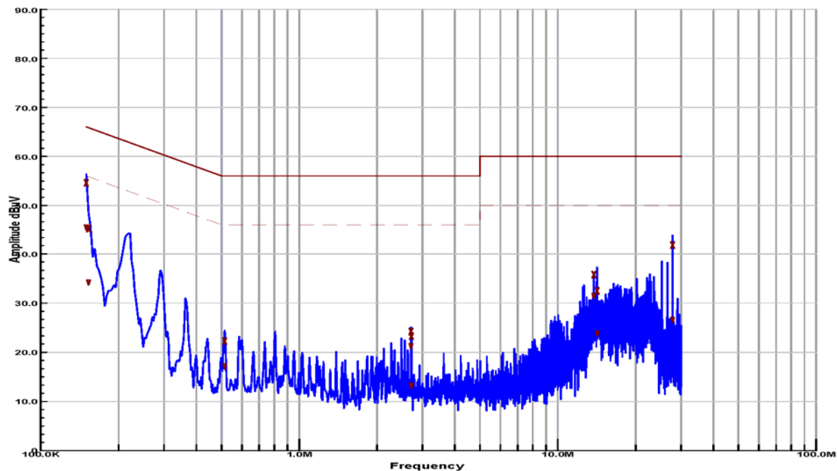
Line (火線)
