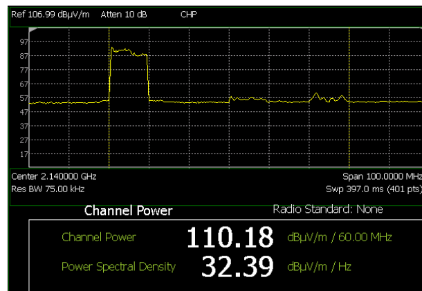
Fig. A3.j 2,1 GHz band, Average: 110,18 dBμV/m k.o.m. 0,32 V/m
