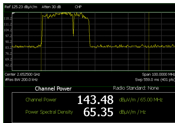
Fig. A3.k 2,6 GHz band, MaxHold: 143,48 dBμV/m k.o.m. 14,93 V/m
