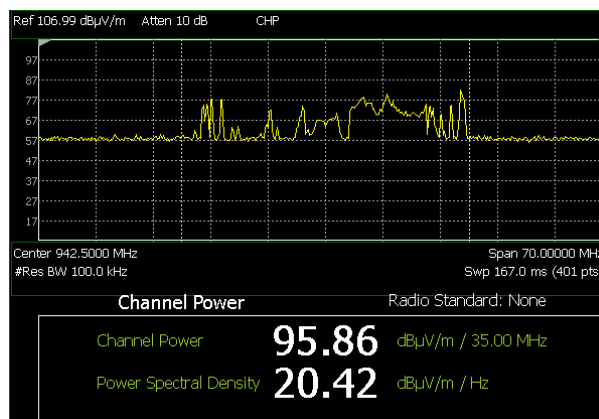
Fig. A3.e 900 MHz band, Maxhold: 95,86 dBμV/m k.o.m. 0,62 V/m
