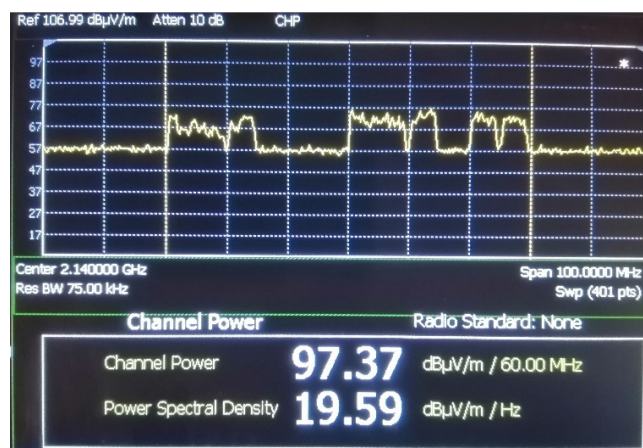
Fig. A1.e 2,1 GHz band: 97,37 dBμV/m k.o.m. 0,074 V/m
