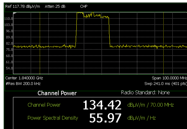
Fig. A3.g 1,8 GHz band, Maxhold: 134,42 dBμV/m k.o.m. 5,26 V/m
