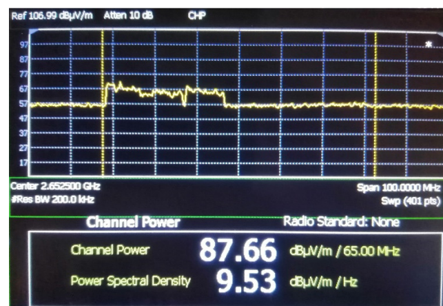
Fig. A1.f 2,6 GHz band: 87,66 dBμV/m k.o.m. 0,024 V/m
