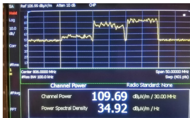
Fig. A2.b 800 MHz band: 109,69 dBμV/m k.o.m. 0,30 V/m
