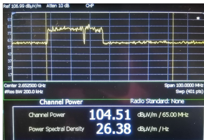
Fig. A2.f 2,6 GHz band: 104,51 dBμV/m k.o.m. 0,17 V/m
