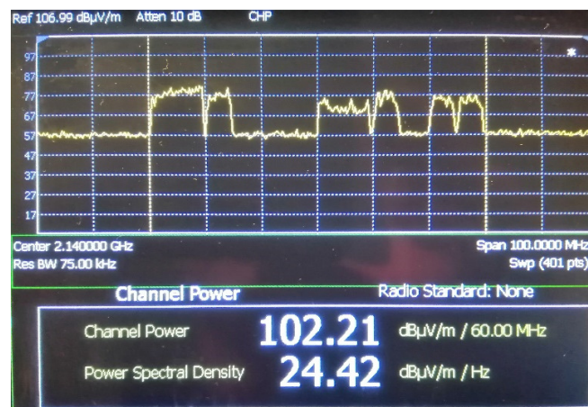
Fig. A2.e 2,1 GHz band: 102,21 dBμV/m k.o.m. 0,13 V/m
