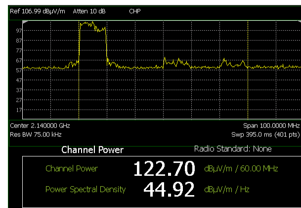
Fig. A3.i 2,1 GHz band, MaxHold: 122,70 dBμV/m k.o.m. 1,36 V/m
