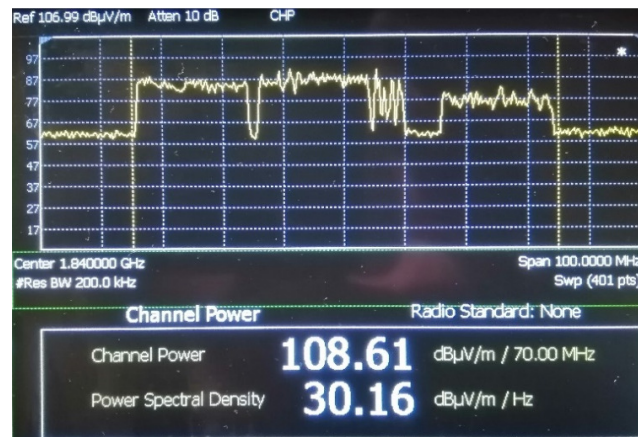
Fig. A2.d 1,8 GHz band: 108,61 dBμV/m k.o.m. 0,27 V/m
