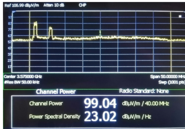
Fig. A2.a 3,5 GHz band: 99,04 dBμV/m k.o.m. 0,089 V/m
