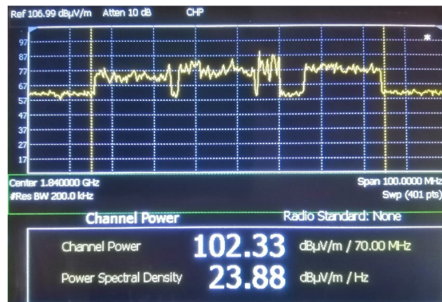
Fig. A1.d 1,8 GHz band: 102,33 dBμV/m k.o.m. 0,13 V/m
