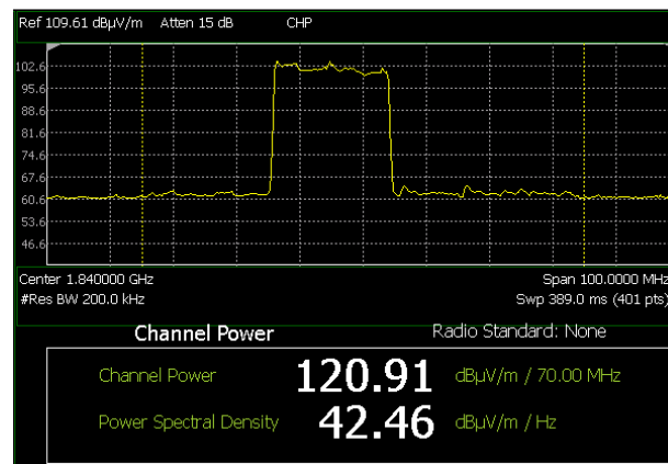
Fig. A3.h 1,8 GHz band, Average: 120,91 dBμV/m k.o.m. 1,11 V/m
