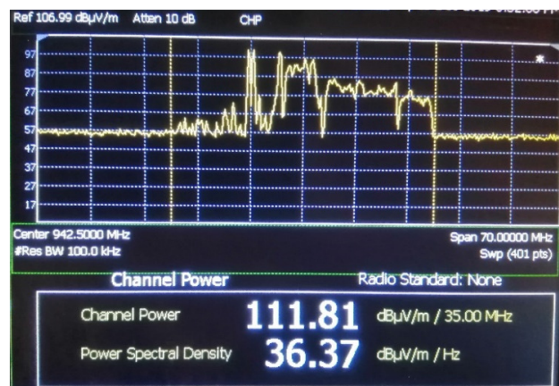
Fig. A2.c 900 MHz band: 111,81 dBμV/m k.o.m. 0,39 V/m
