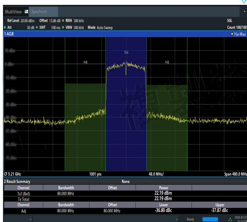
NTVN-11AC80SISO-Ant2-5210-PASS
