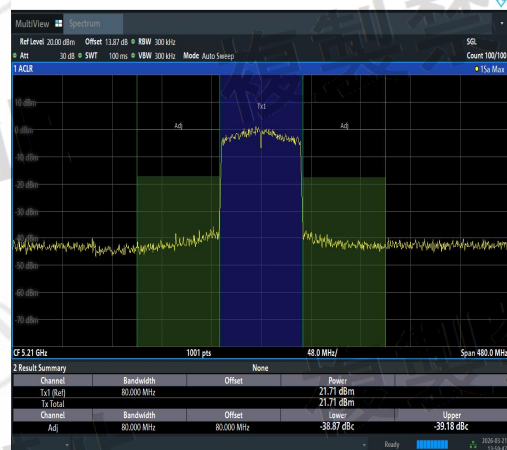
NTVN-11AC80SISO-Ant3-5210-PASS
