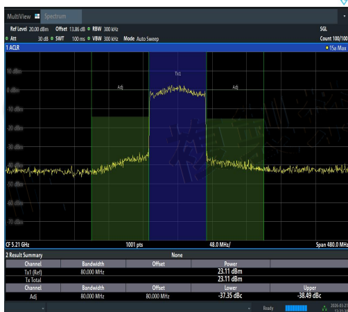
NTVN-11AX80SISO-Ant2-5210-PASS
