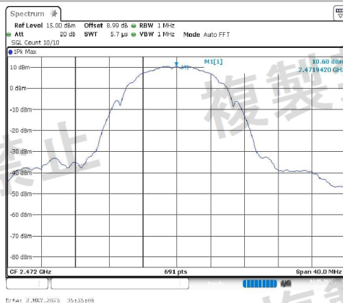
NTVN-11B-Ant1-2472-PASS
