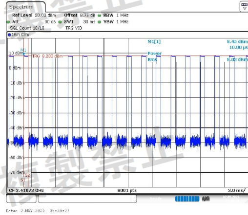
NTVN-11B-Ant1-2412-PASS
