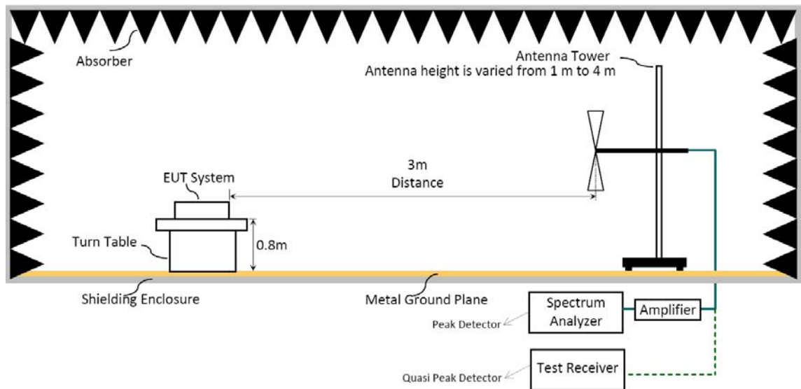
圖 1: 量測頻率低於 1GHz 之測試配置(No.1 3m Semi Anechoic Chamber)
