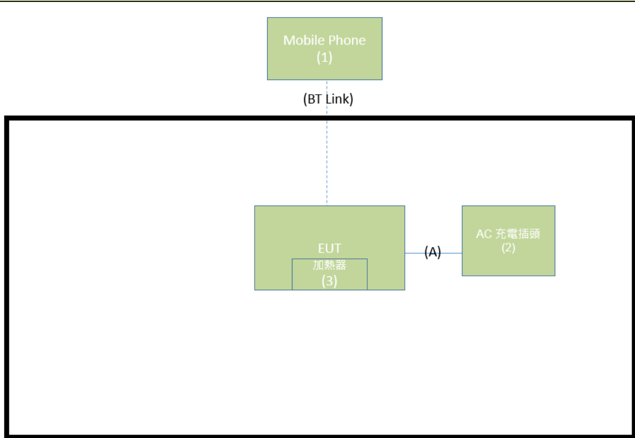
待測物測試配置圖 (Mode 3)
