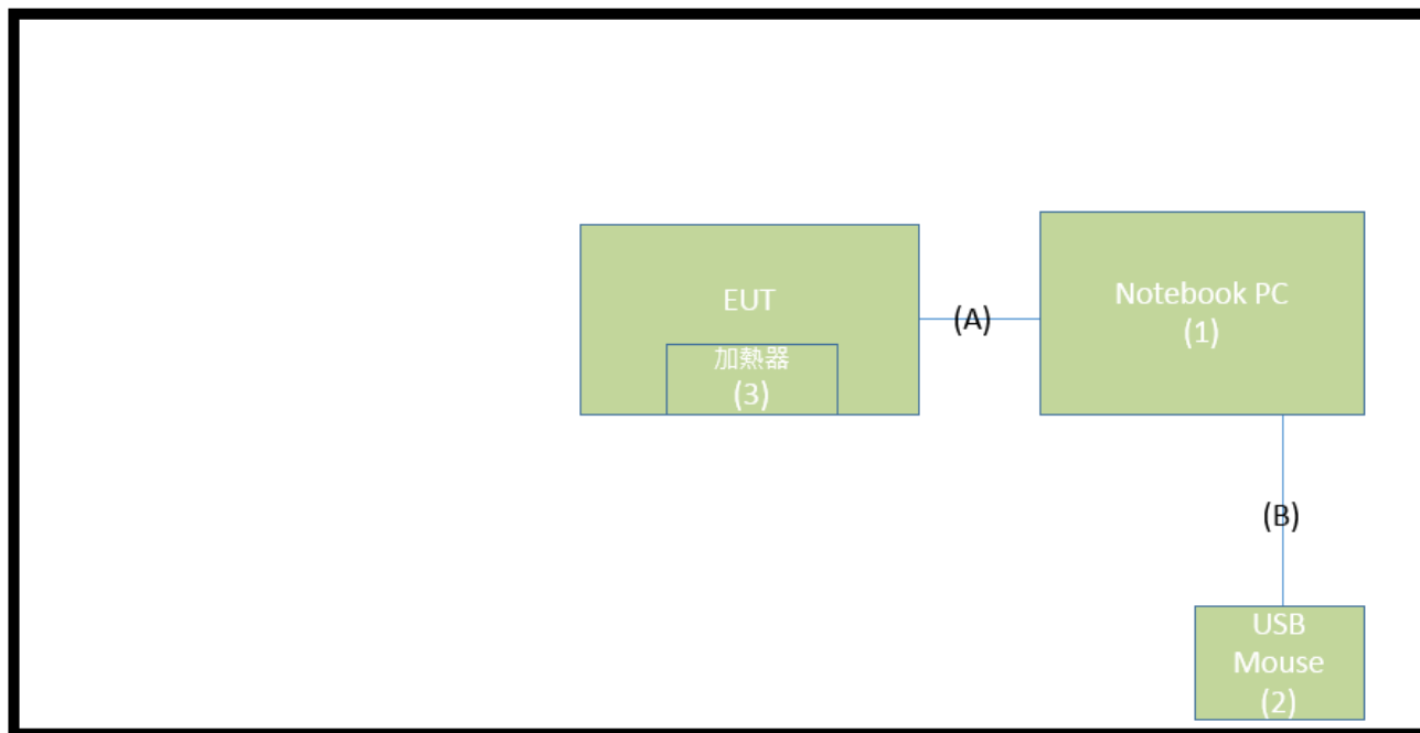
待測物測試配置圖 (Mode 1/2)
