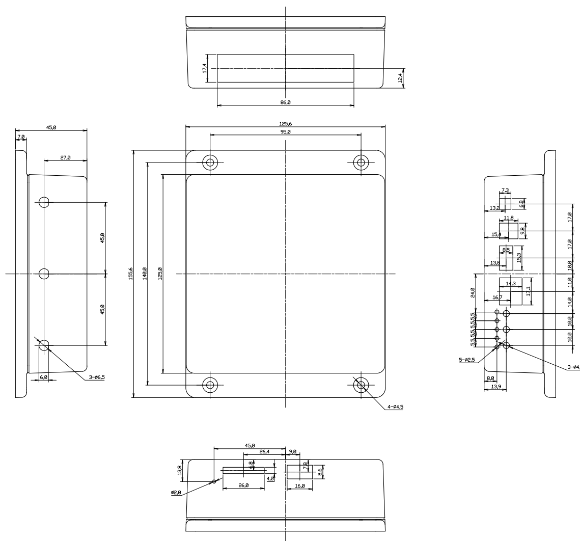
図 19.6 Armadillo-IoT ゲートウェイ スタンダードモデルの筐体 形状図
