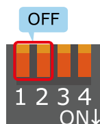
図 18.25 全二重で使用する場合の設定スイッチ(SW1)の状態
