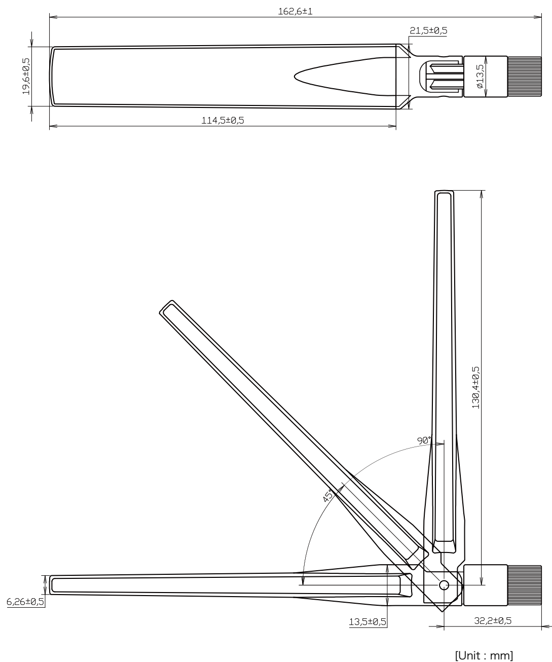
図 19.4 アンテナ形状
