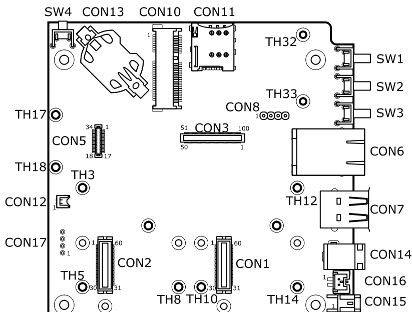
図 16.1 Armadillo-IoT ゲートウェイ ベースボード インターフェースレイアウト(A 面)
