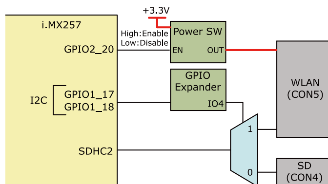
図 14.1 WLAN インターフェース(CON5)周辺の構成
