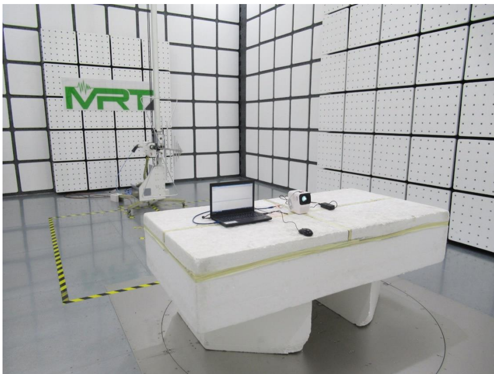
輻射測試 Above 1GHz
