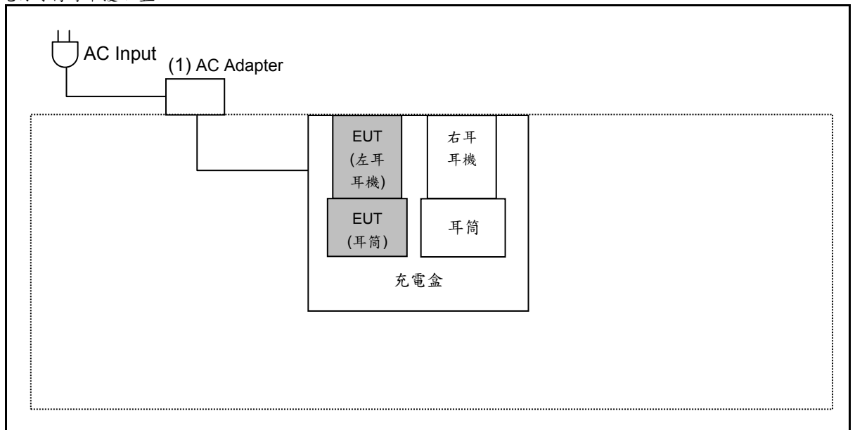
電源線傳導干擾配置
